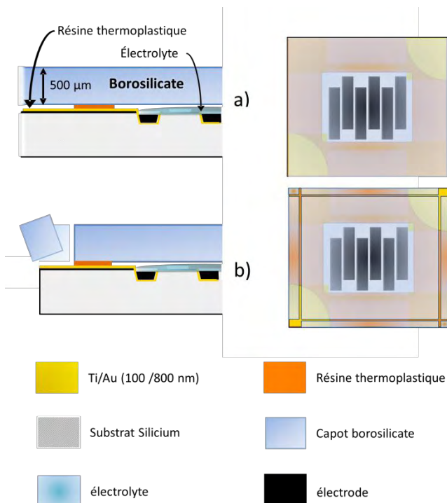
Fig. 64 – procédé d'encapsulation de l'électrolyte liquide : a) dépôt de résine photosensible et thermoplastique sur un substrat transparent (borosilicate ou silice fondue), b) découpe en 2 temps
