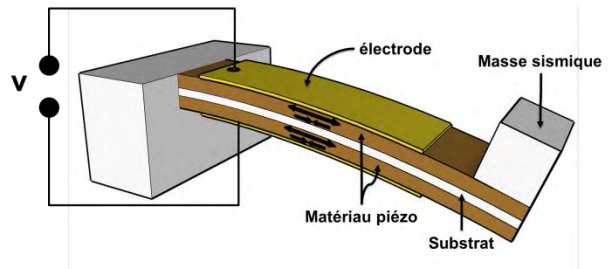
Fig. 19 – dispositif de récupération d'énergie à partir de vibrations au format poutre bimorphe.
