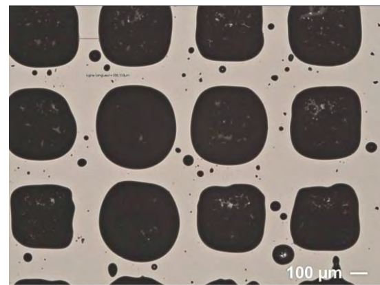
Fig. 60 – image microscope d'un dépôt sur \text{Si}_3\text{N}_4 plan par sérigraphie à travers des ouvertures carrées dans un masque métallique. La pâte est composée de charbon actif lié par du PVDF dans de l'éthylène glycol.
