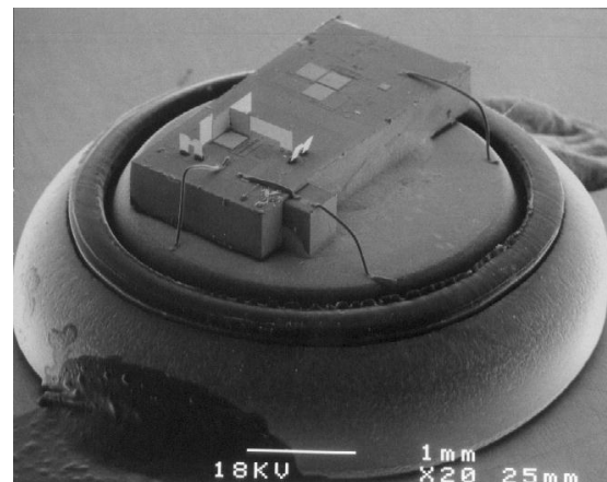
Fig. 3 – Smart Dust monté sur une pile bouton Lithium : l'alimentation électrique occupe 80 % du volume du système. [5]
