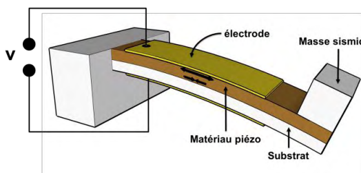
Fig. 18–dispositif de récupération d'énergie à partir de vibrations au format poutre unimorphe.
