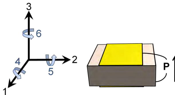
Fig. 16—Indices utilisés dans le formalisme piézoélectrique, pour un élément dont la polarisation a la direction et le sens de P .
