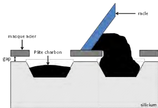
Fig. 59 – schéma du dépôt de pâte par sérigraphie avec masque acier.
