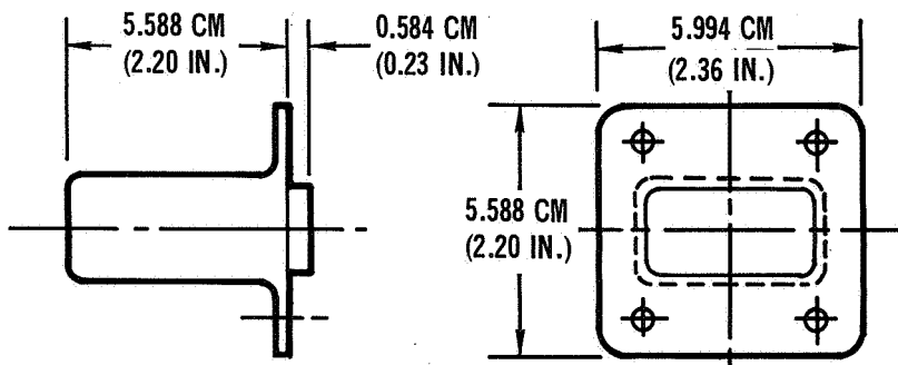
C-Band Linear Slot Antenna
