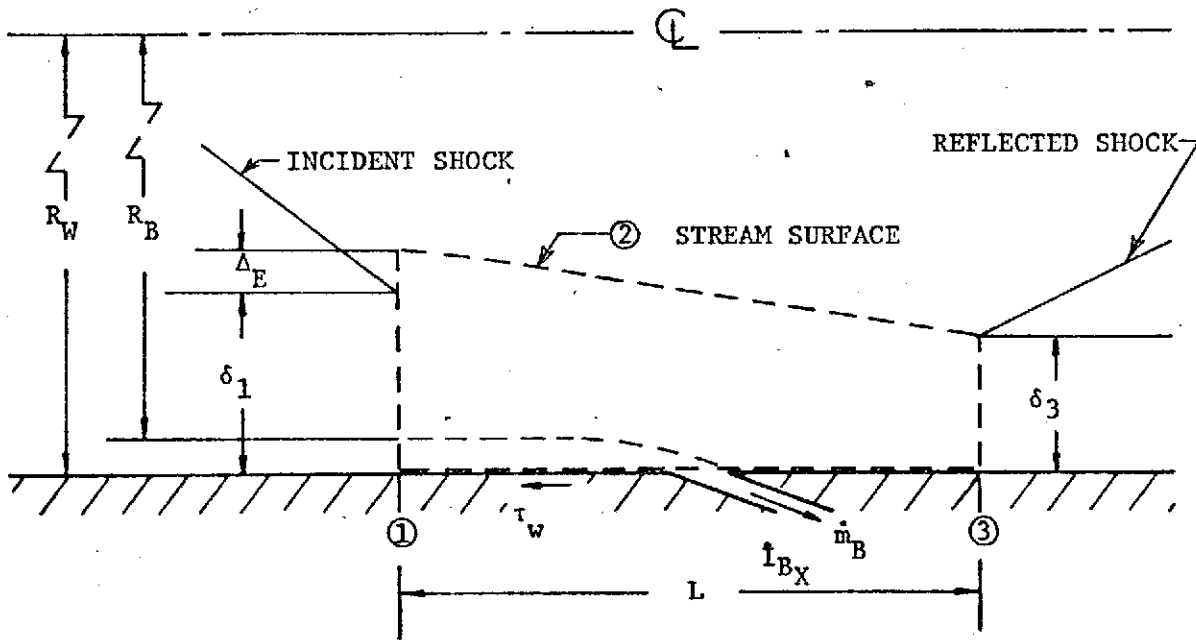
(b) SLOT BLEED
