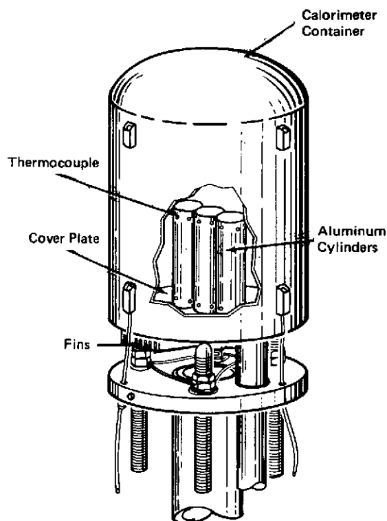
Calorimeter
