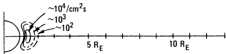
a. PROTON FLUX, E > 30 MeV
