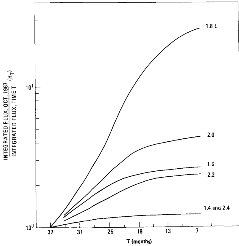
d. E > 500 keV
