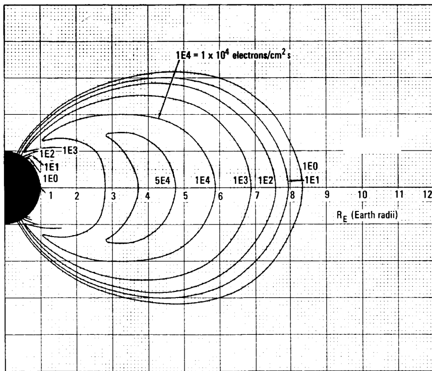
c. E > 3.0 MeV
