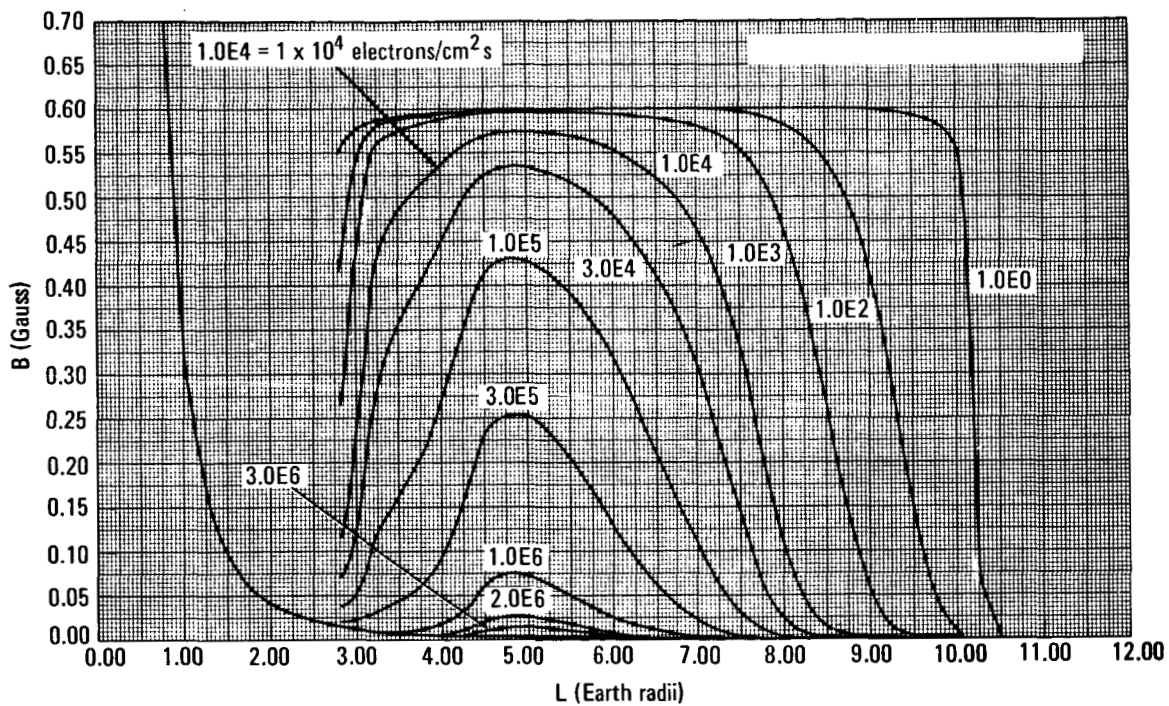
a. E > 0.5 MeV
