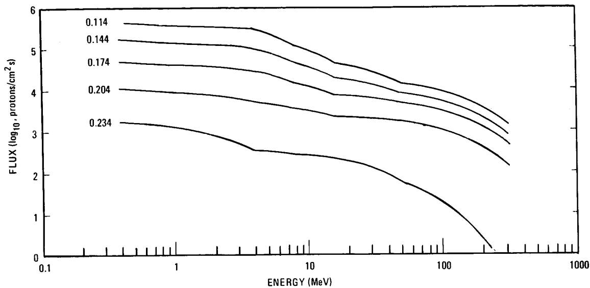
a. 0.114 to 0.234 Gauss
