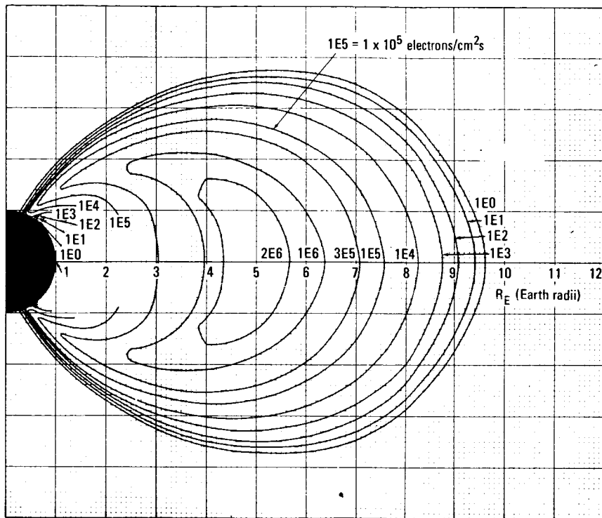
b. E > 1.0 MeV
