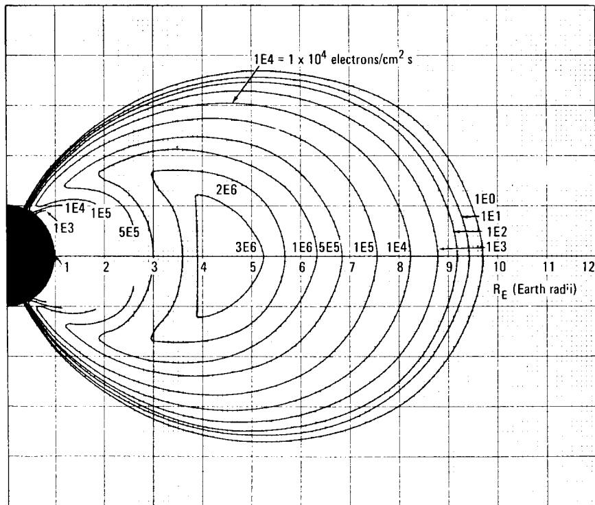
b. E > 1.0 \text{ MeV}
