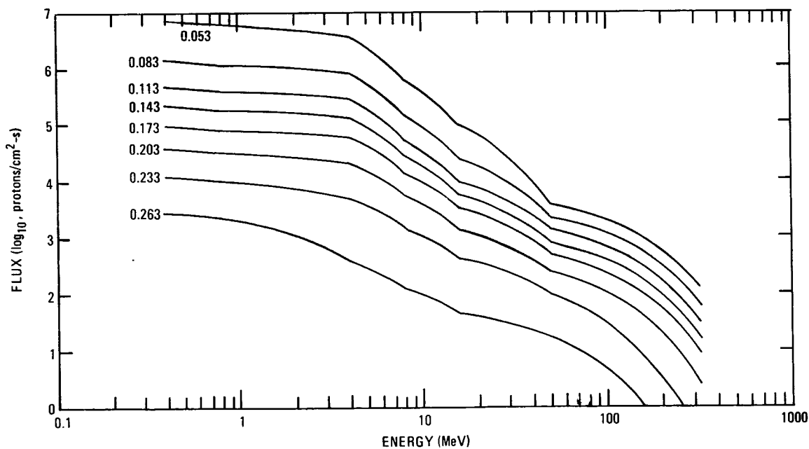
b. 0.053 to 0.263 Gauss
