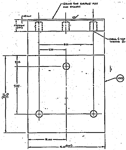
-070 ASSY (1 REQD) SCALE: 1/2
