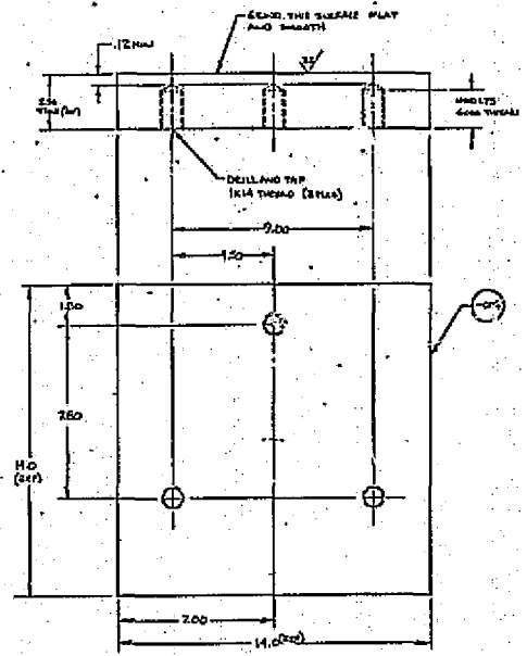
-060 ASSY (1 REQD) SCALE: 1/2
