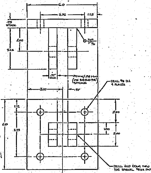
-050 ASSY 2 REQD MATL: ASTM A36 STEEL SCALE: FULL
