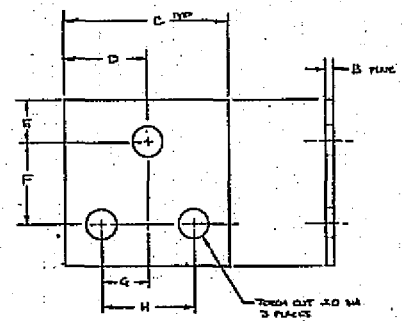
MATL: ASTM A36 STEEL SCALE: NONE
