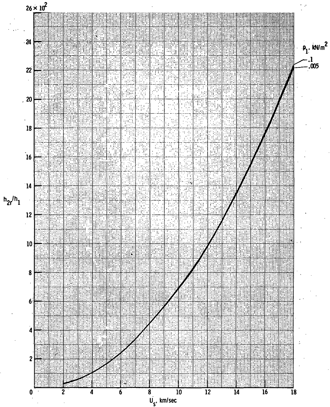
(d) Enthalpy h_{2r}/h_1 .
