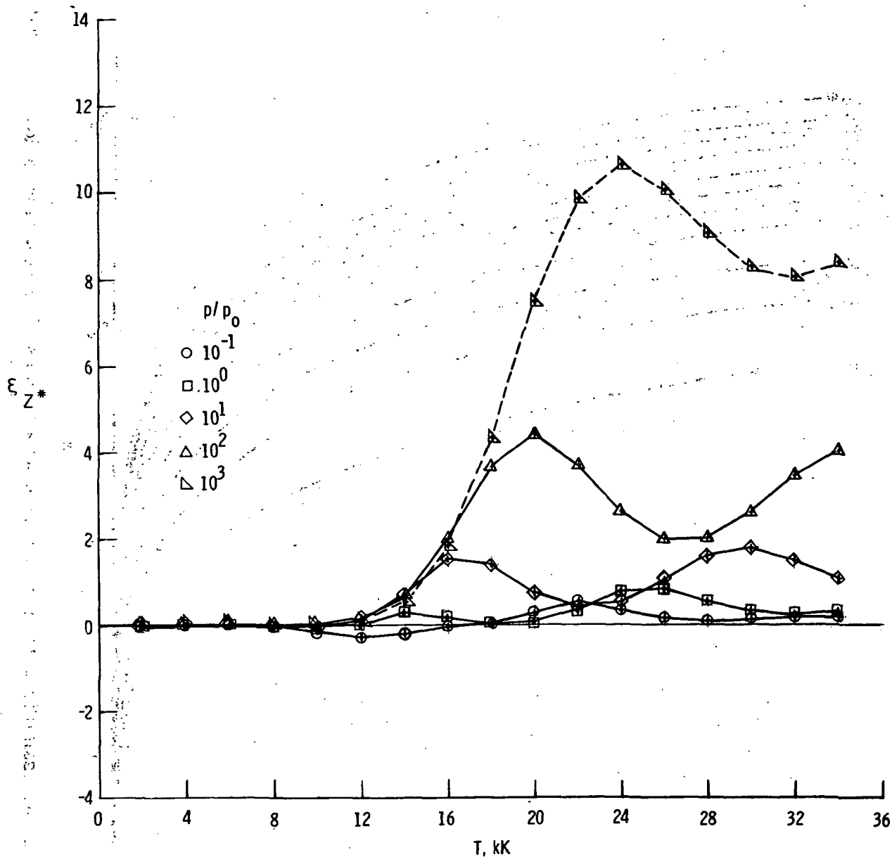
(d) Molecular-weight ratio Z^* .
