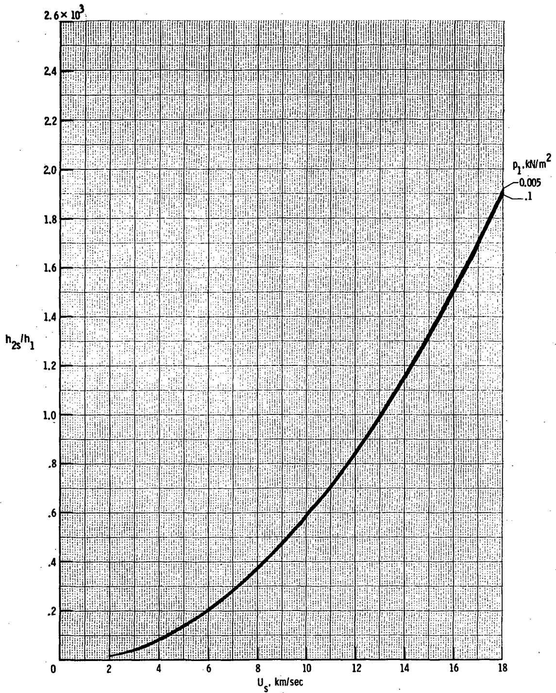
(d) Enthalpy h_{2s}/h_1 .
