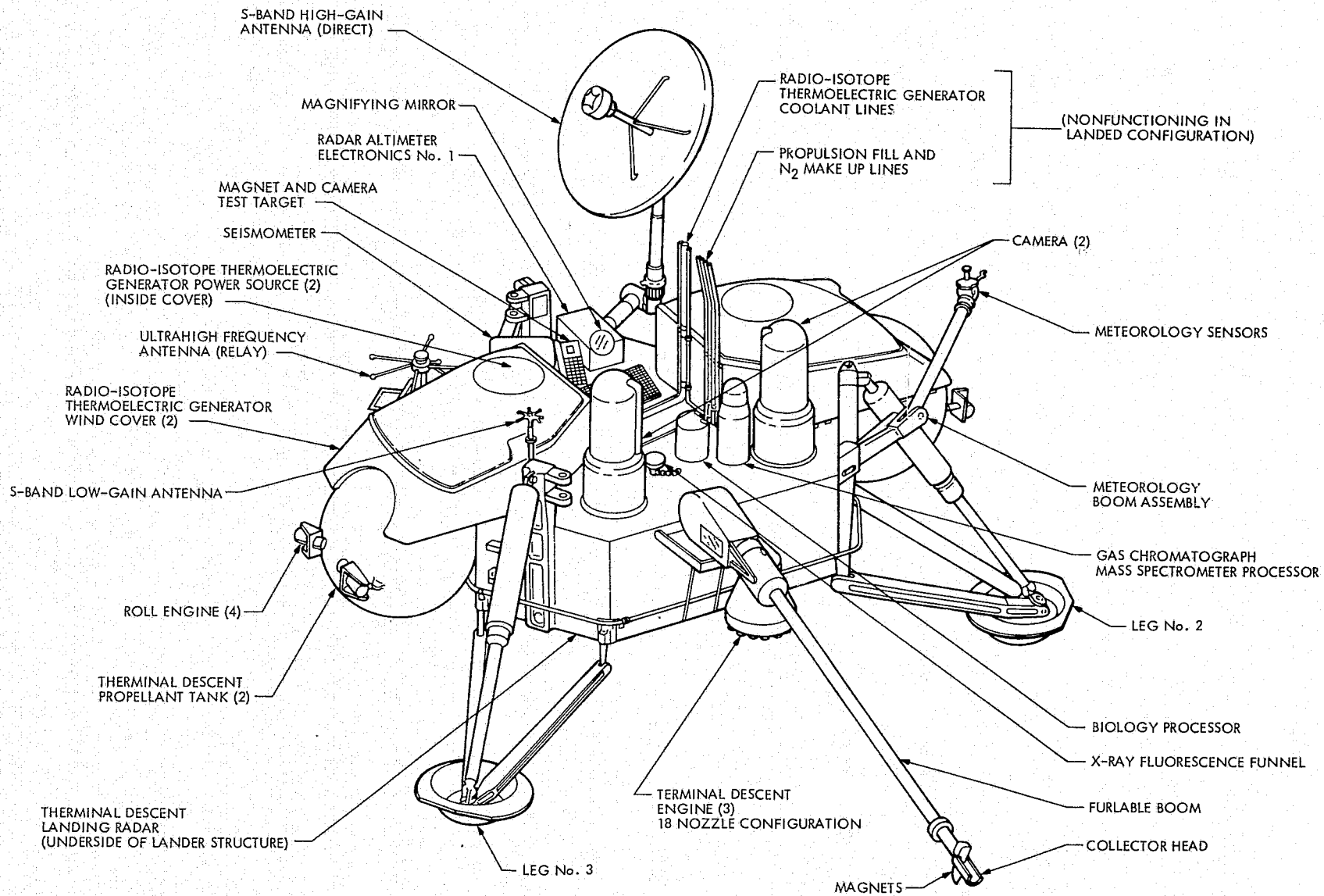
Fig. 8. Viking Lander
