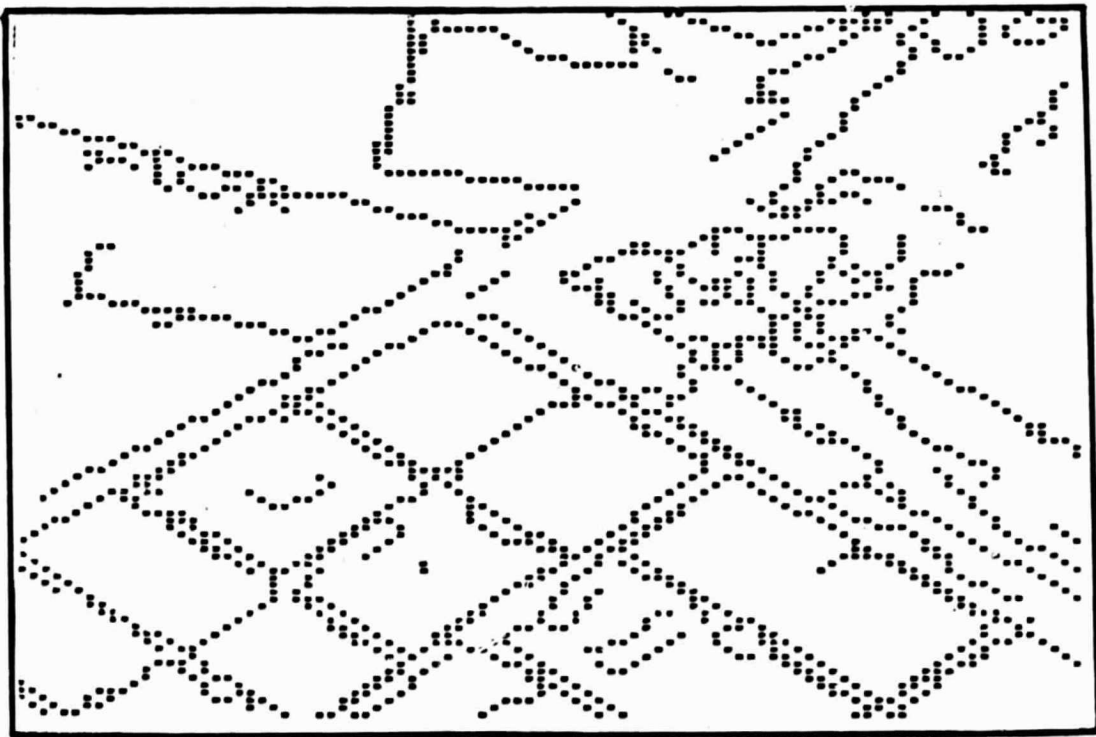
Fig. 6 - Edge detection
