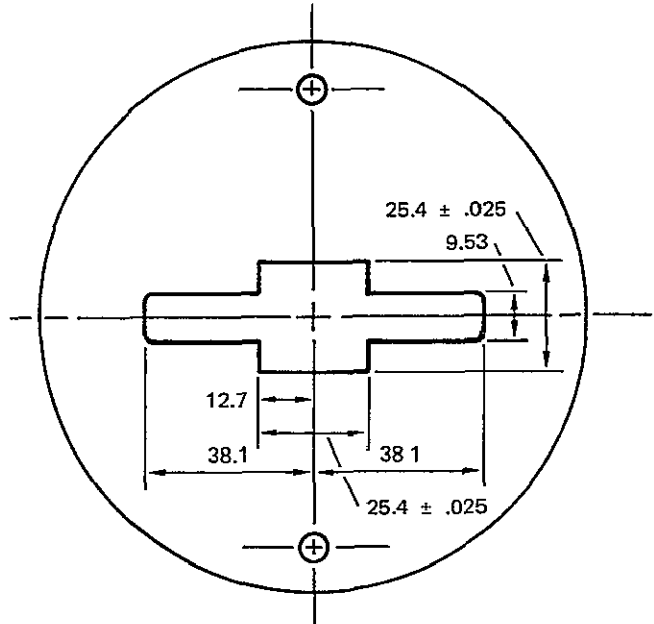
(d) RECEPTACLE 3
