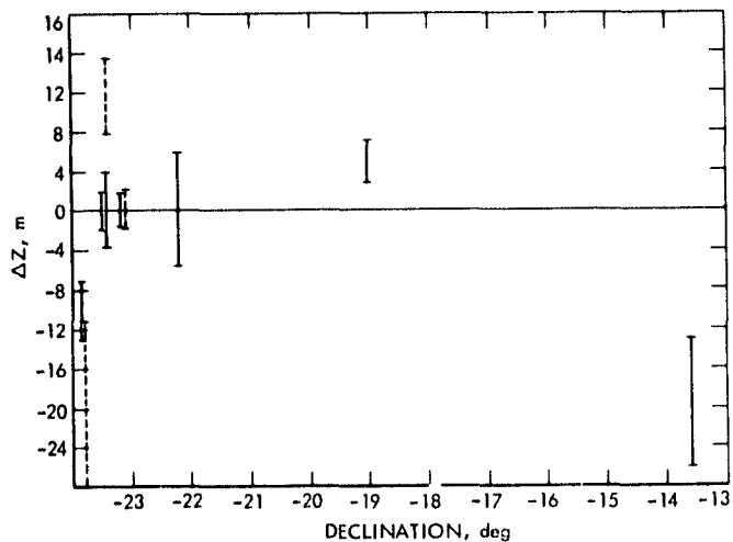
Fig. 10. \Delta Z estimates for DSS 43—DSS 14 baseline
