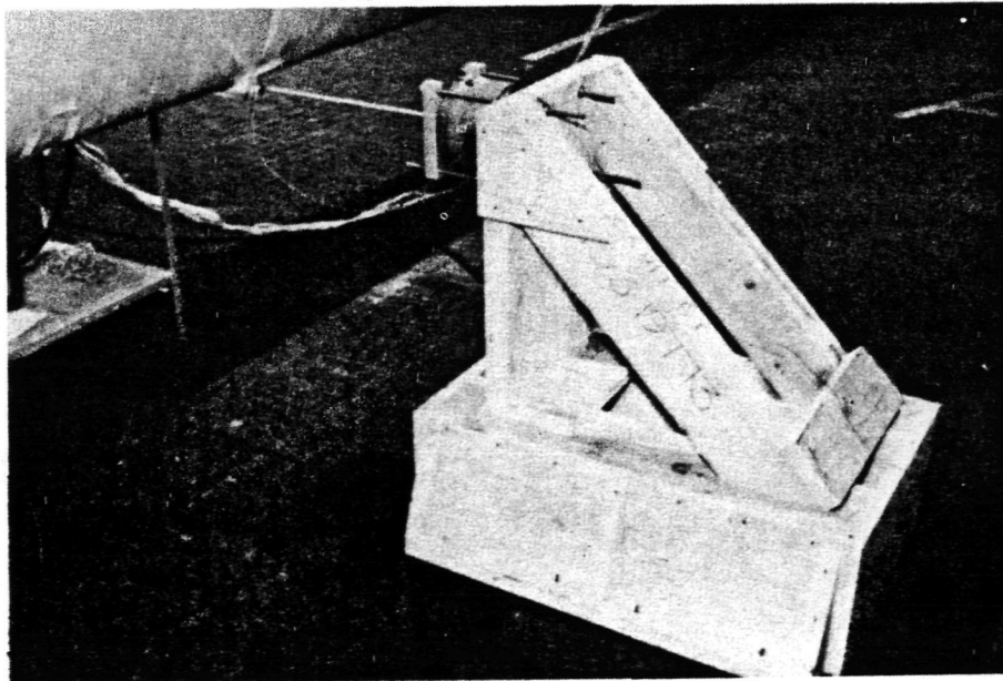
B. FLATWISE MODE
