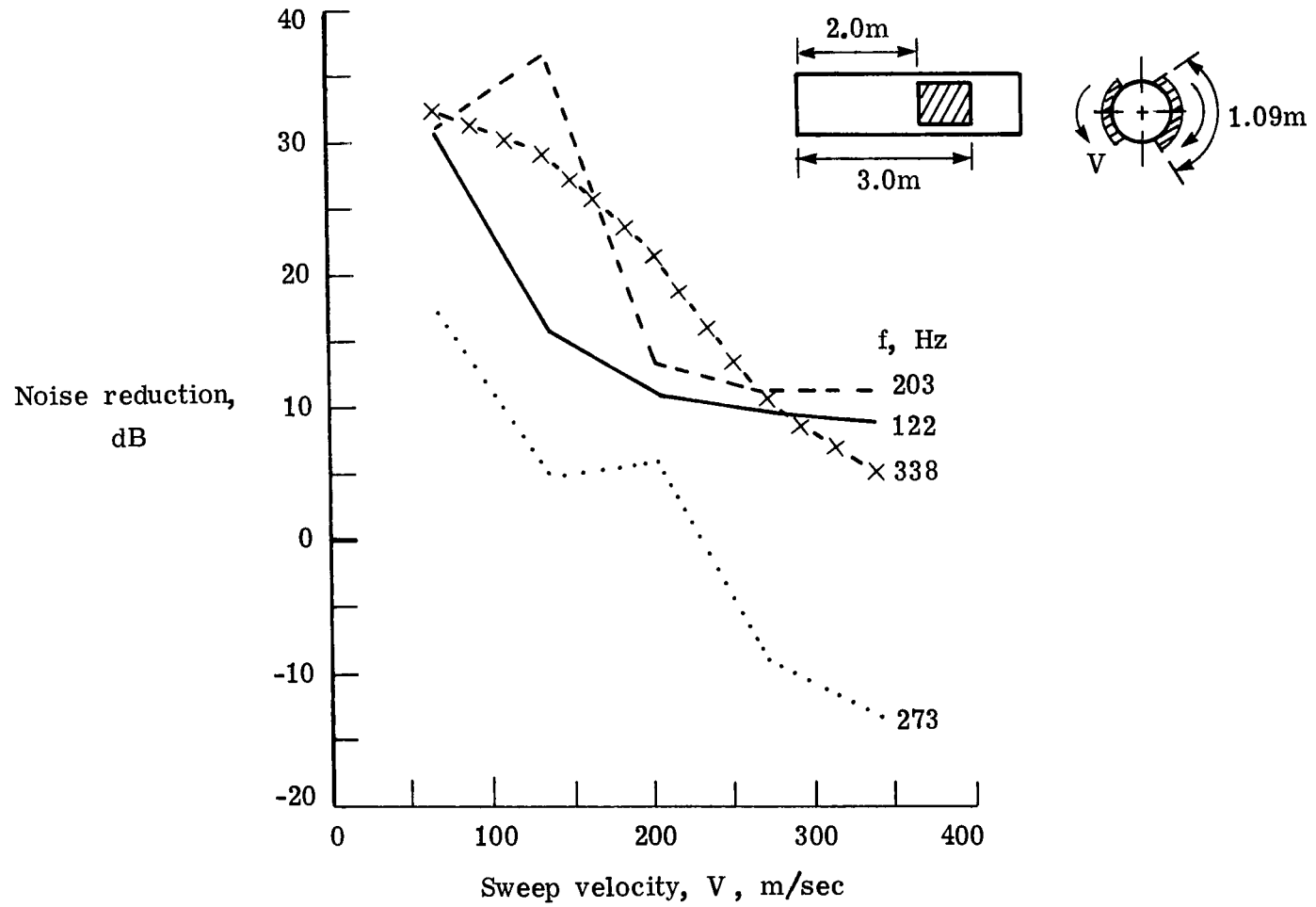
(b) Fuselage 2.
