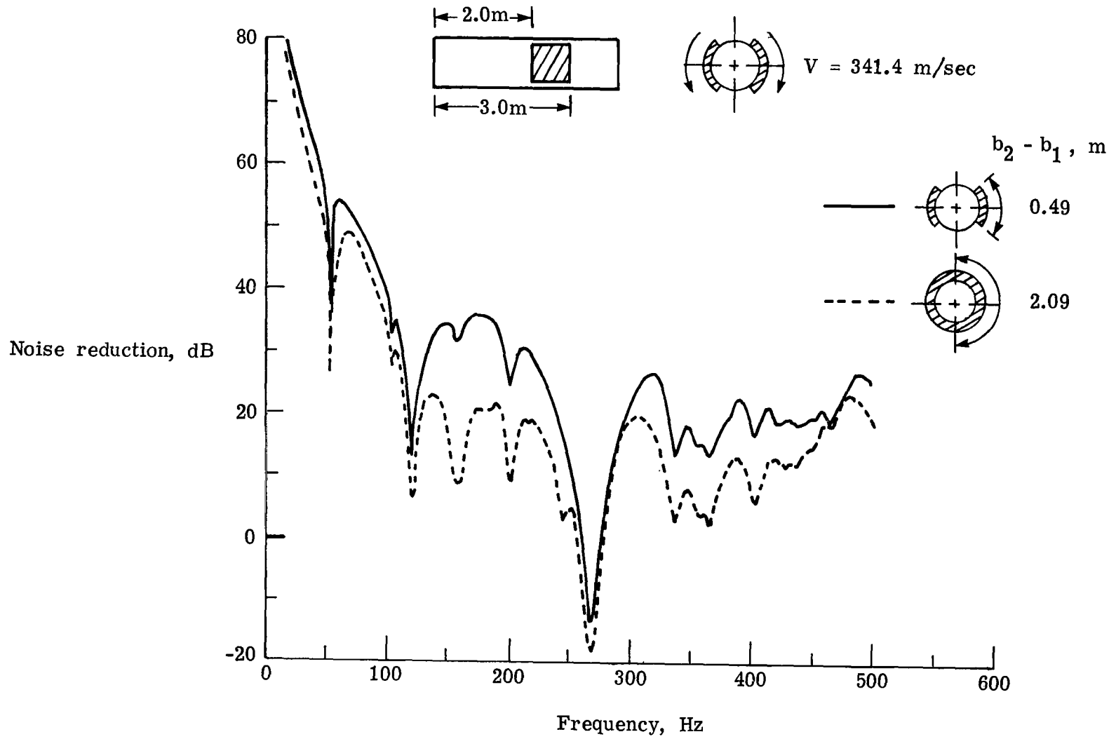
(b) Fuselage 2.
