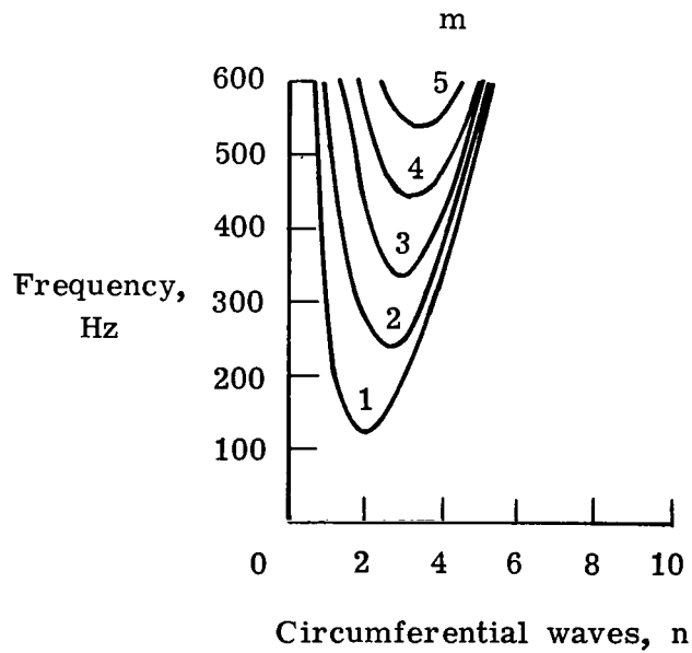
(b) Fuselage 2.
