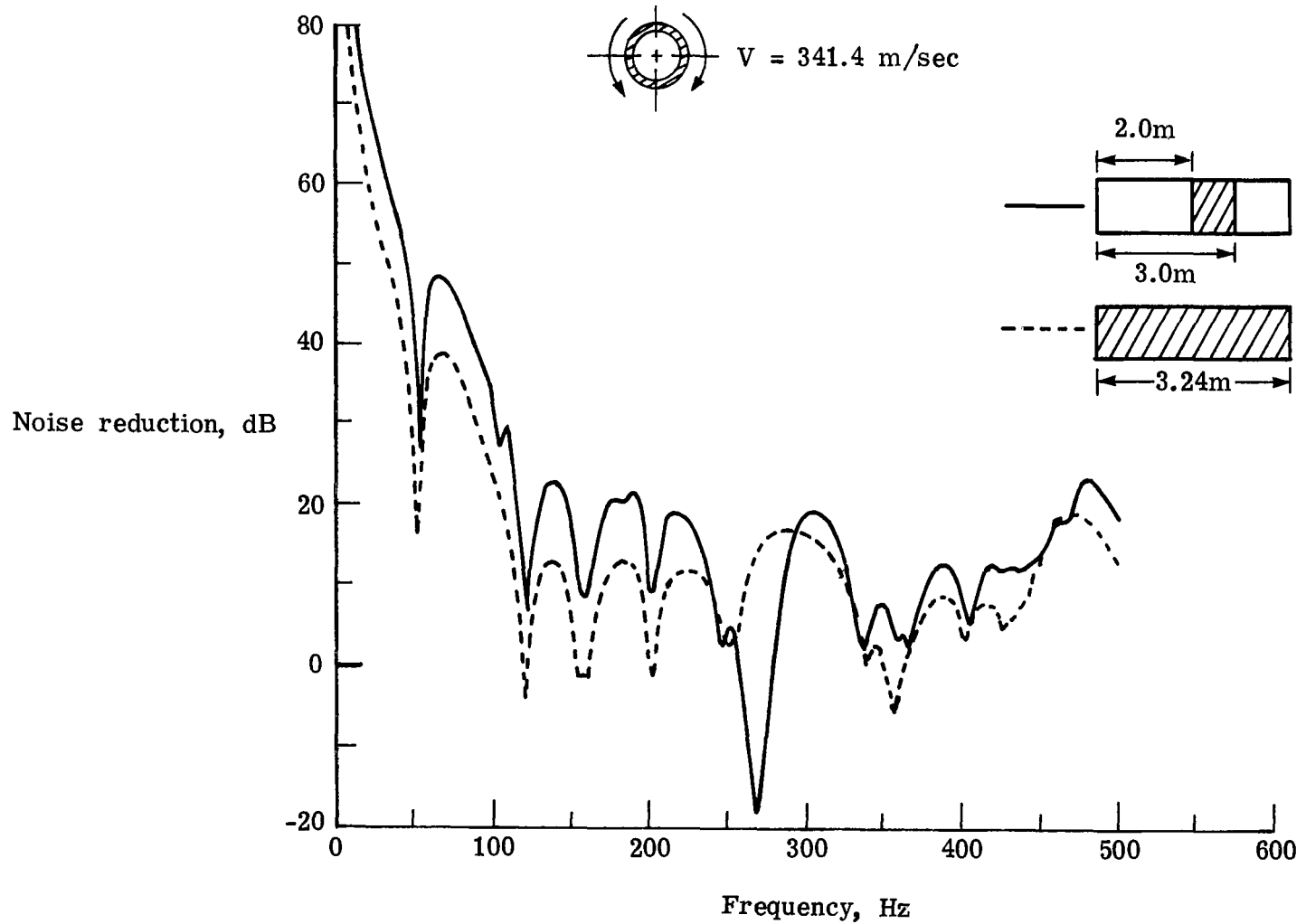
(b) Fuselage 2.
