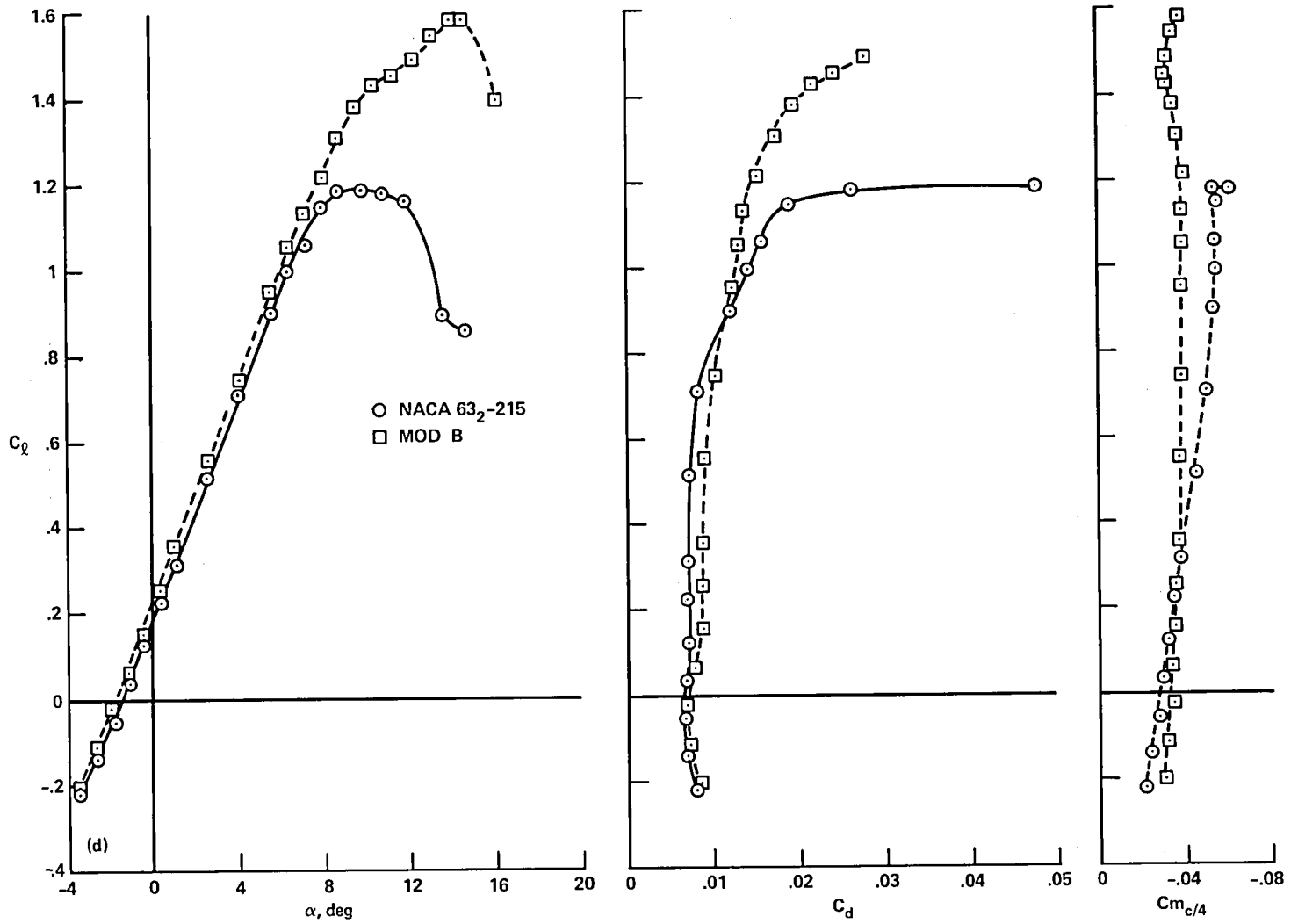
(d) M = 0.3 ; Re = 1.36 \times 10^6
