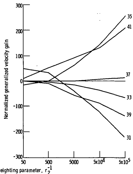
(d) Generalized velocity feedback gains.
