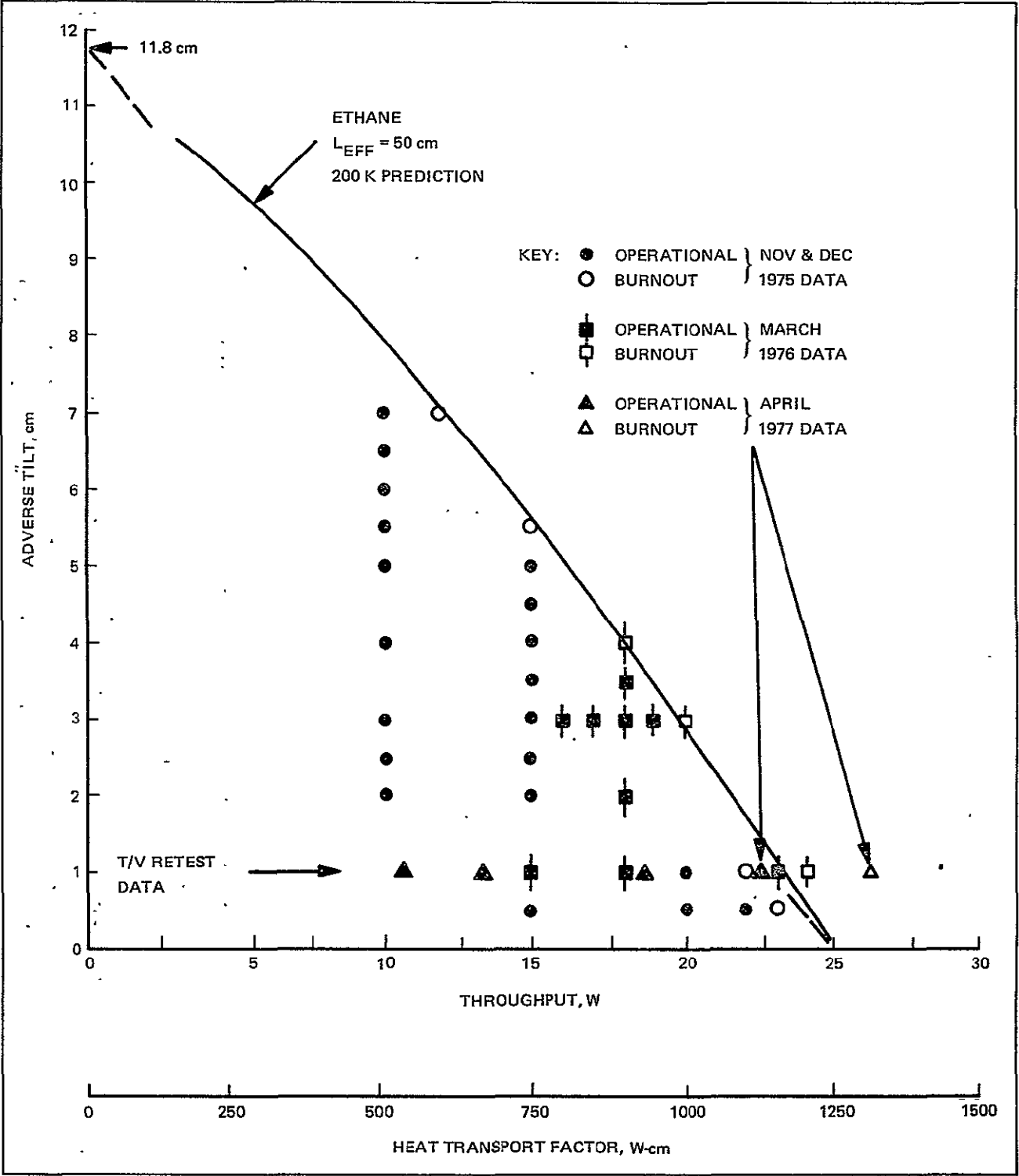
Fig. 5-2 Cryodiode Test Points
