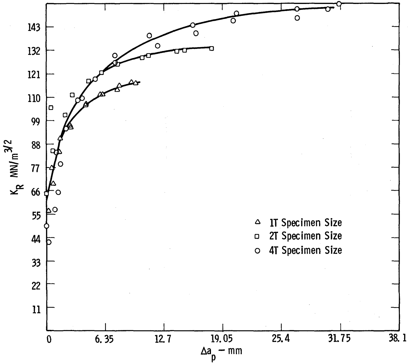
Fig. 3 - 2024-T351
