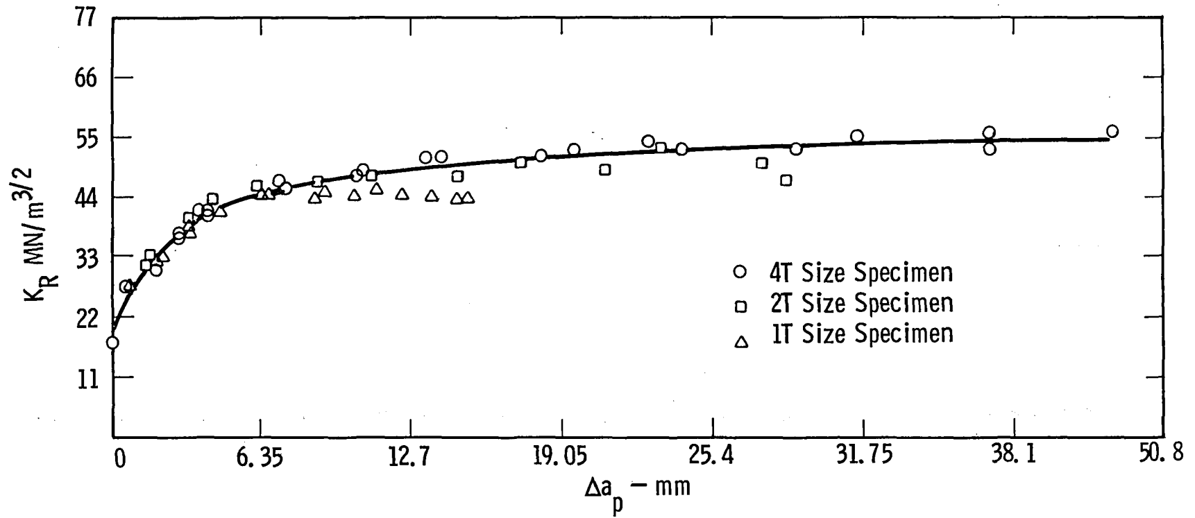
Fig. 5-7075-T651
