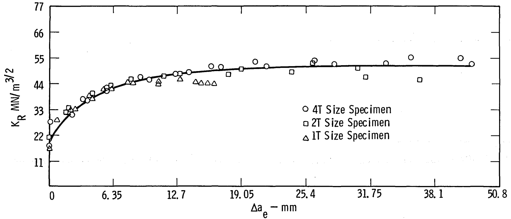
Fig. 4 - 7075 - T651
