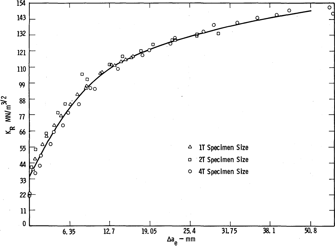
Fig. 2 - 2024-T351
