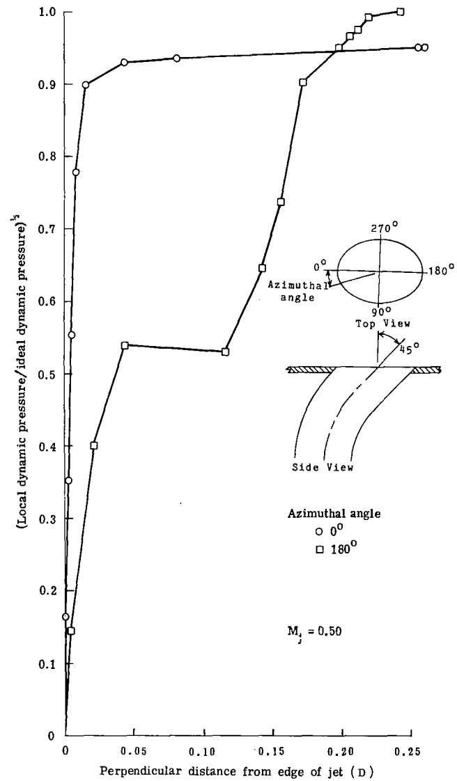
(d) 45° deflection nozzle.
