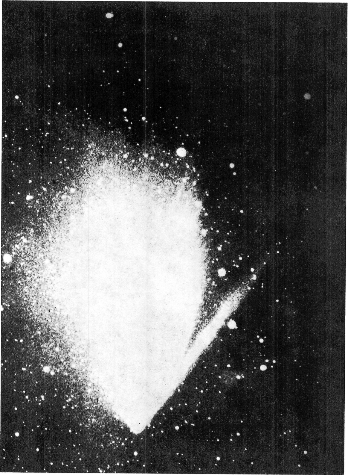
Fig. 1. Comet 1910 I.
