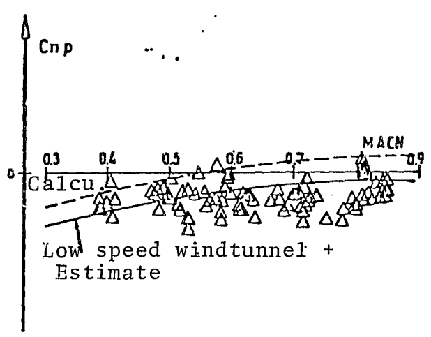
FIG. 18 Yaw Due to Roll
