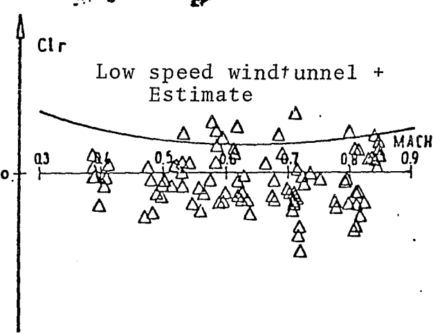
FIG. 19 Roll Due to Yaw
