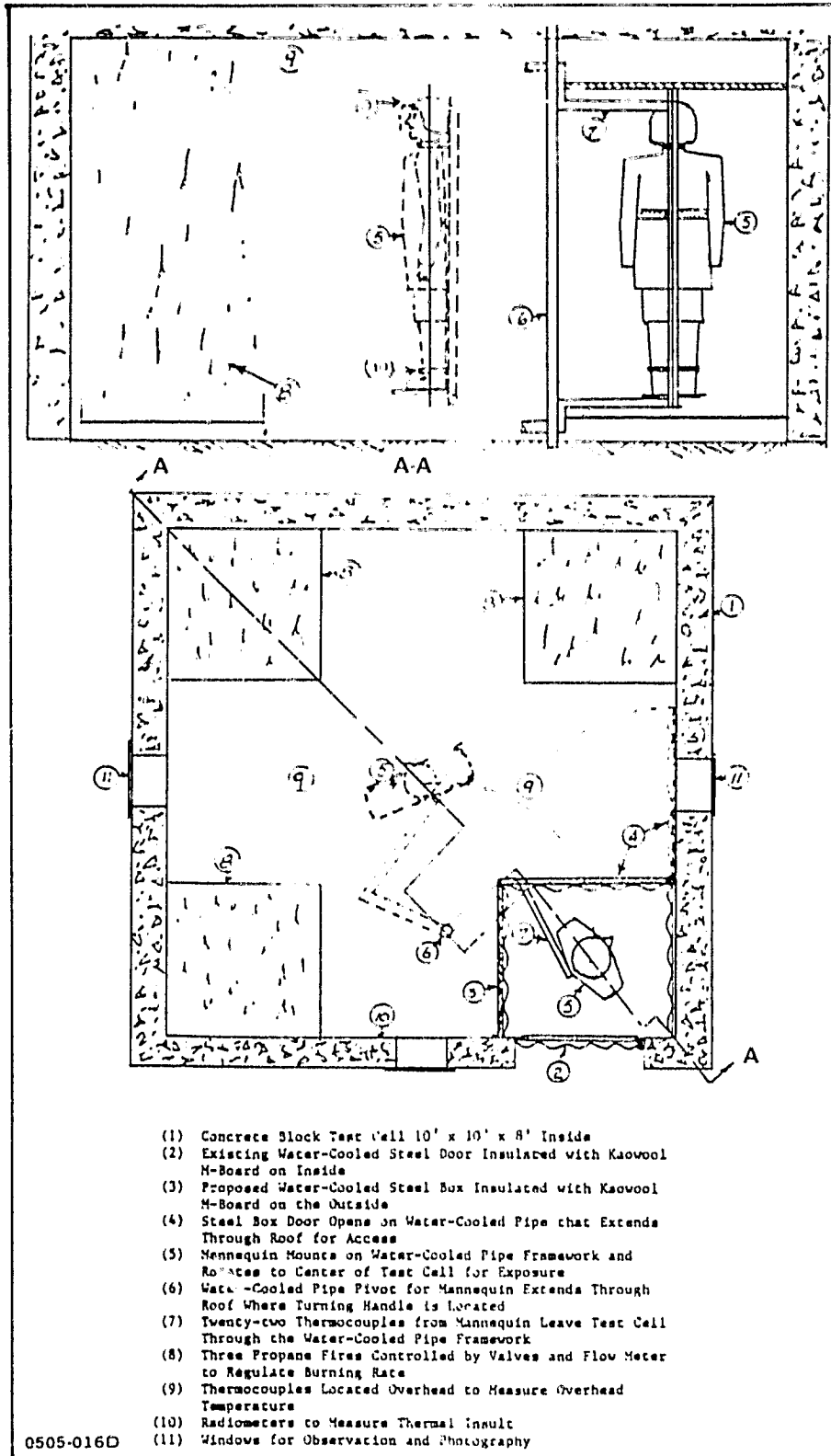
Fig. 4 Test Setup
