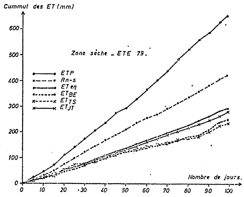
Fig. V - Cumul des valeur d'évaporation sur la série journalière de l'été 79 Z.S.
