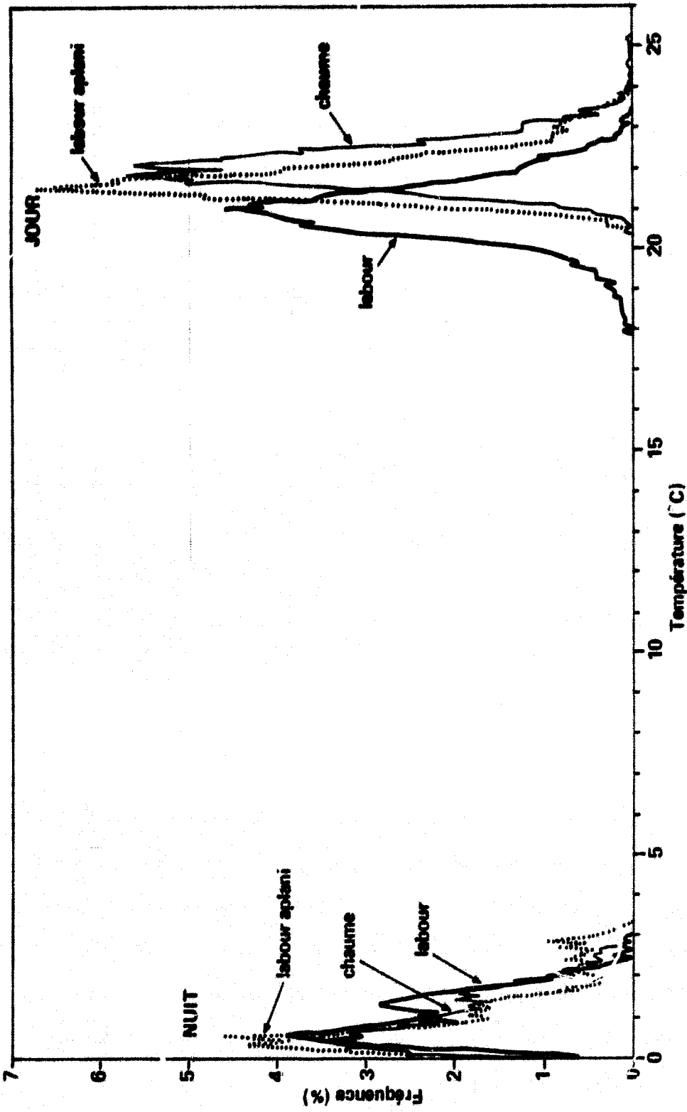
Fig. 9b. Spectres comparés jour et nuit des diverses surfaces de sol (— labour; .....labour aplani; ---- chaume).
