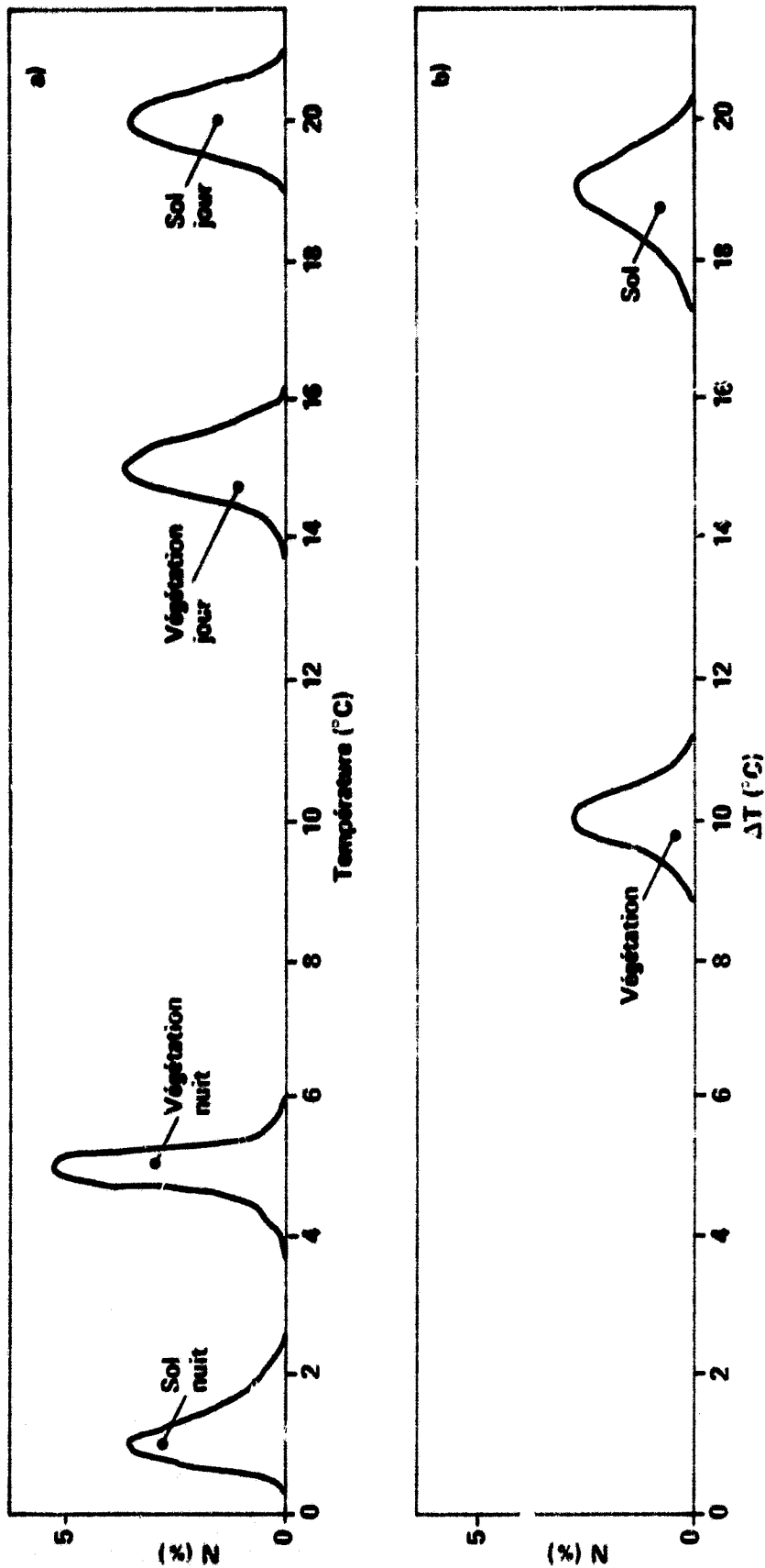
Fig. 10. a) Spectres comparés jour et nuit de deux parcelles contiguës de Maïs (no. 1) et de sol nu (no. 65). b) Spectres de l'écart jour-nuit des températures de la parcelle de Maïs (no. 1) et de sol nu (no. 65).
