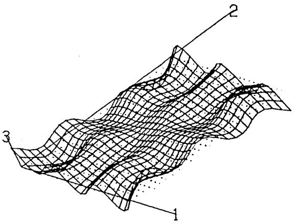
Mode 33 (0.199 Hz)
