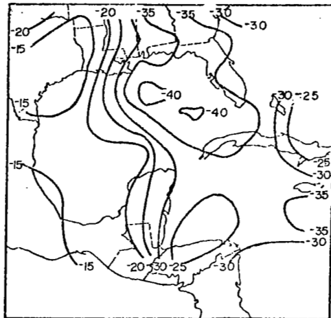
a. Rawinsonde (RW), 500 mb
