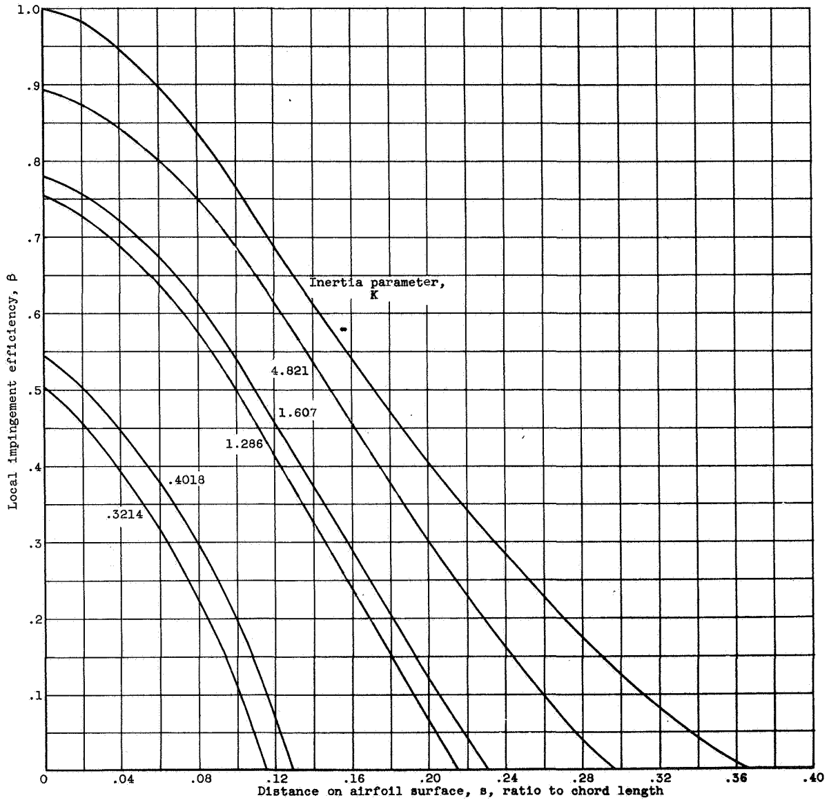
(d) Free-stream Reynolds number, 256.
