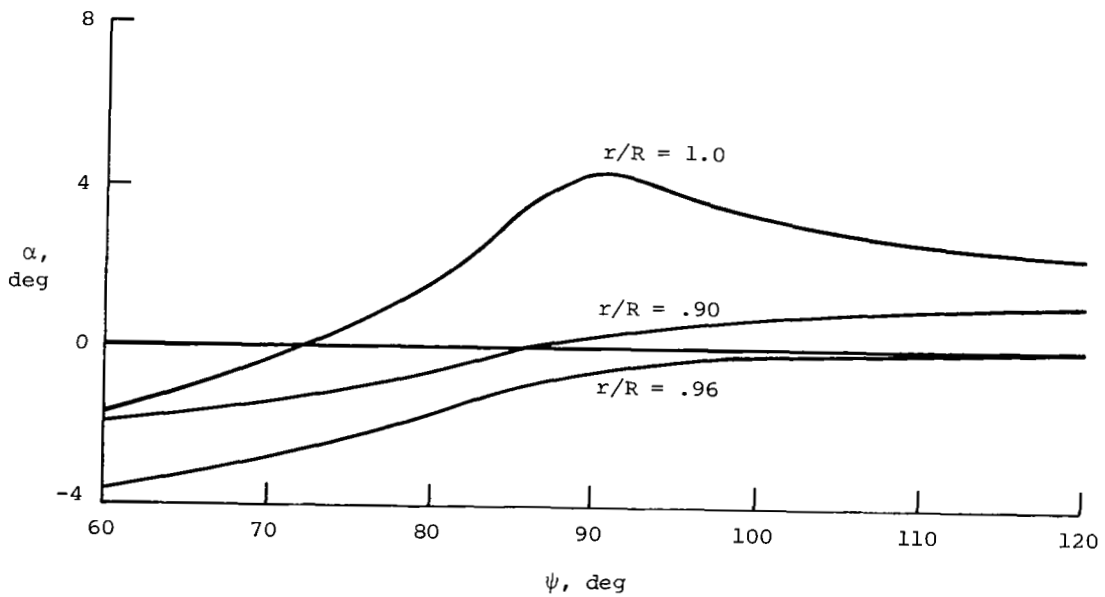
(d) \mu = 0.30 ; C_L/\sigma = 0.08 ; \alpha_s = -4^\circ ; nonuniform inflow.
