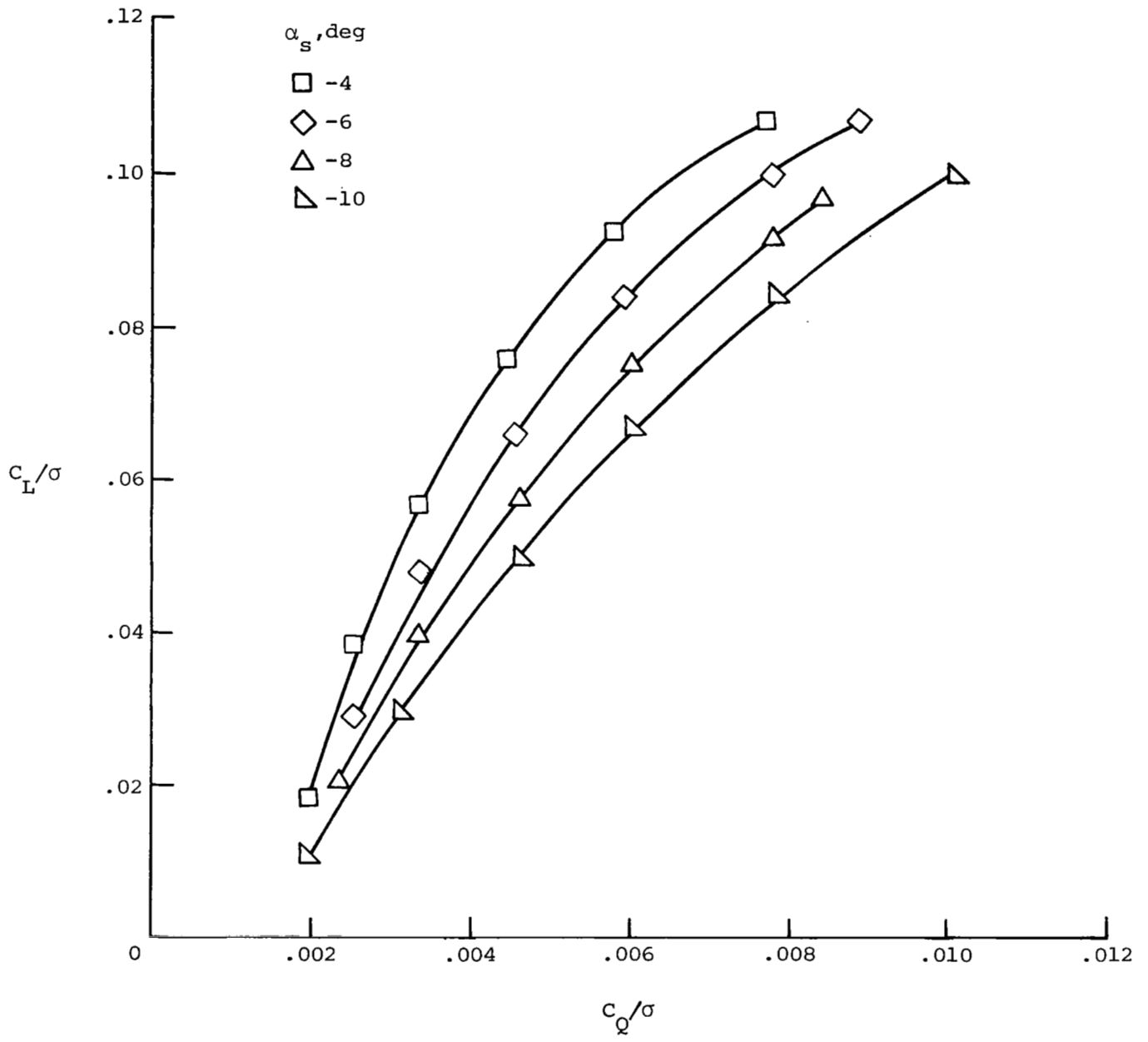
(d) C_L/\sigma versus C_Q/\sigma at \mu = 0.30 .
