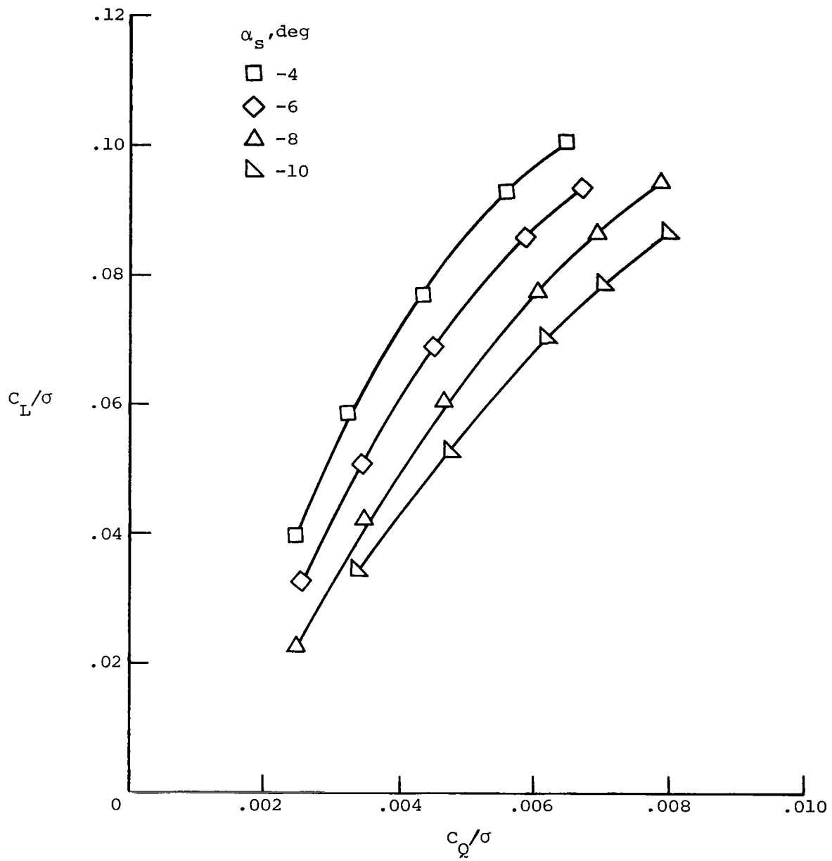
(d) C_L/\sigma versus C_Q/\sigma at \mu = 0.30 .
