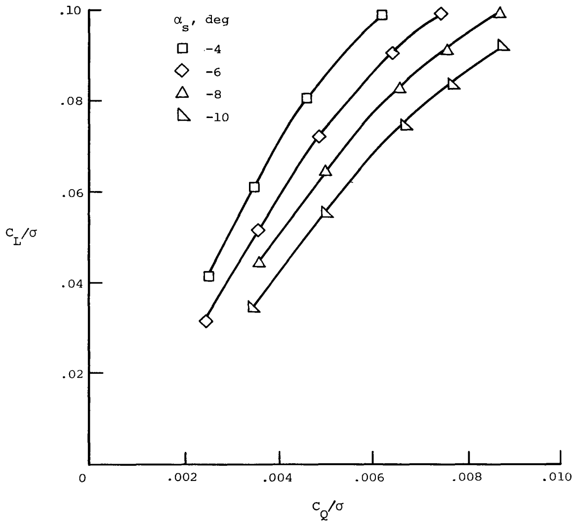
(d) C_L/\sigma versus C_Q/\sigma at \mu = 0.30 .
