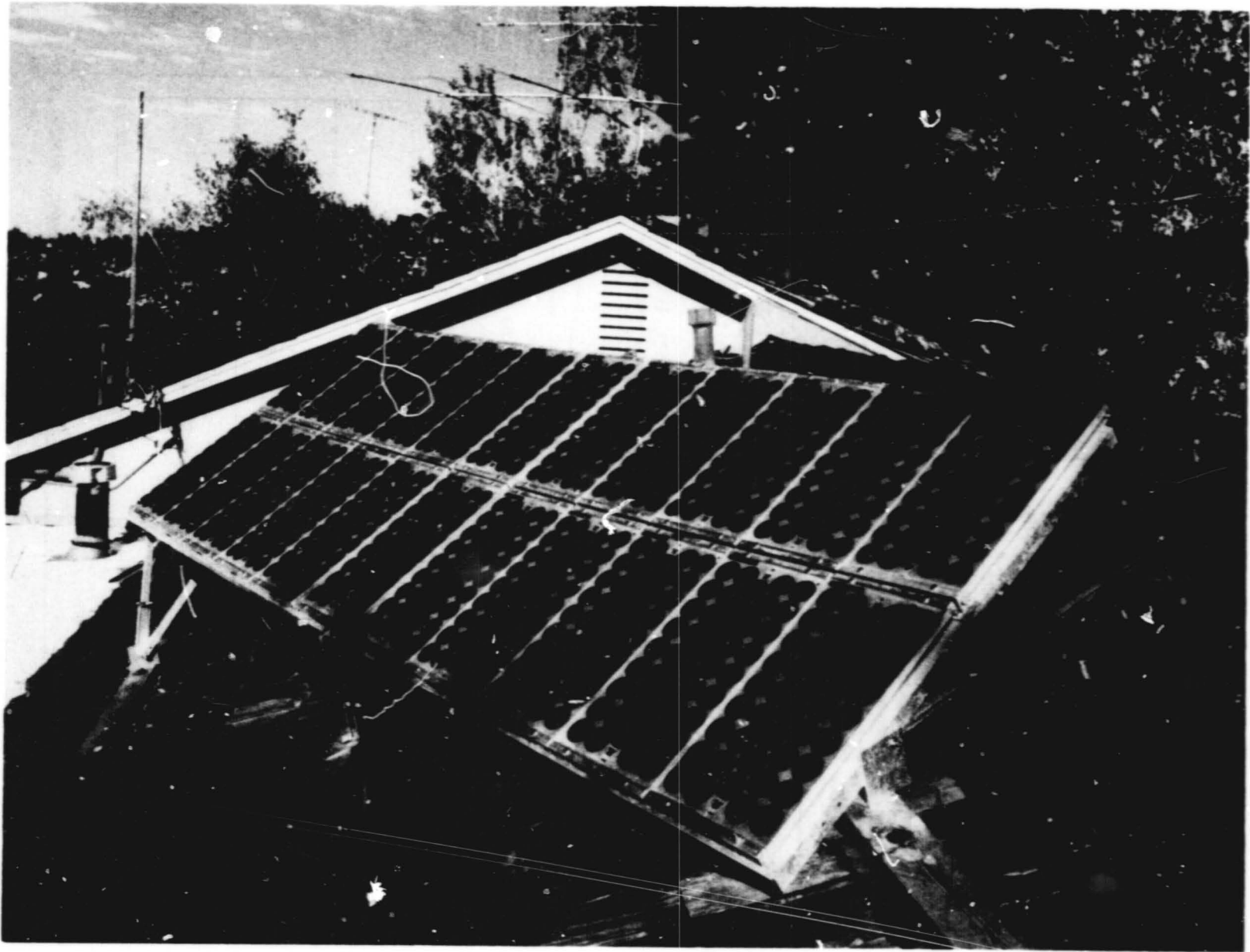
Figure 28. PV Array
