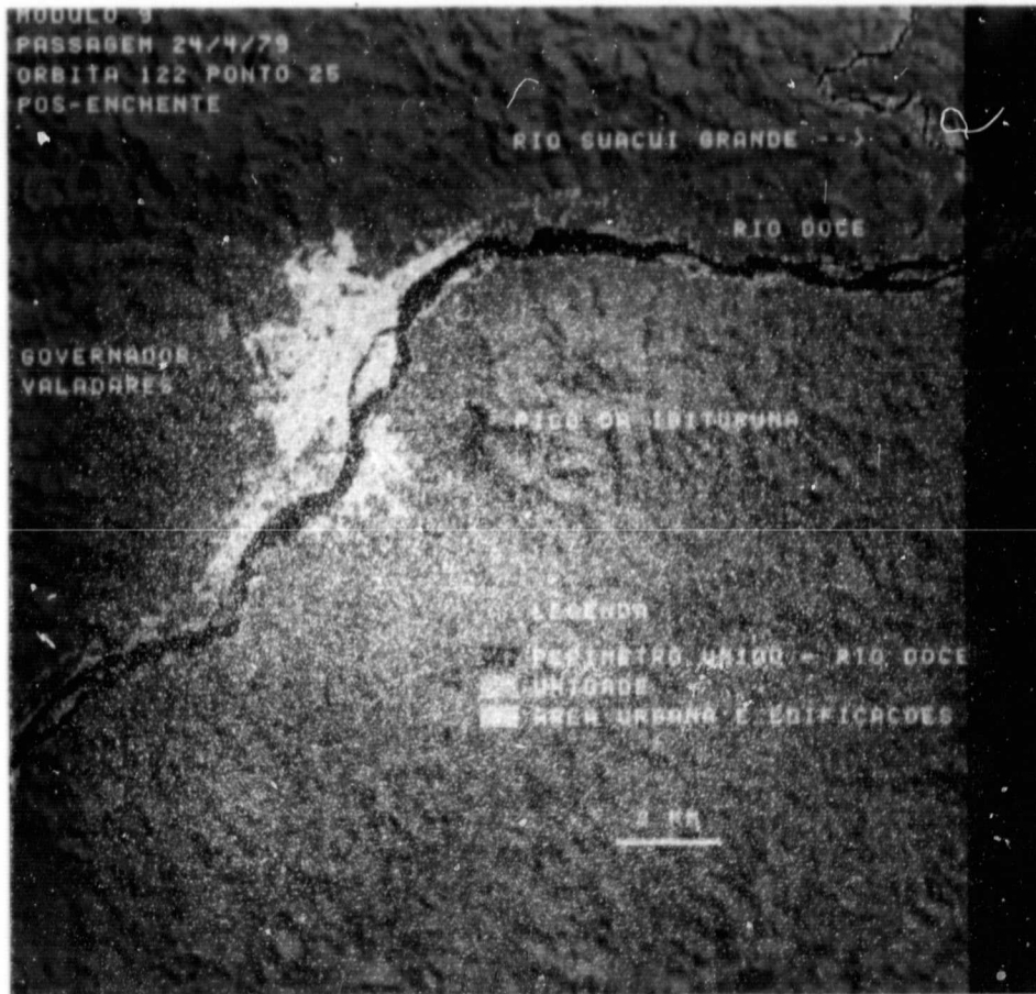
Fig. III.3 - Classificação temática do módulo IX - período de pós-enchente.
