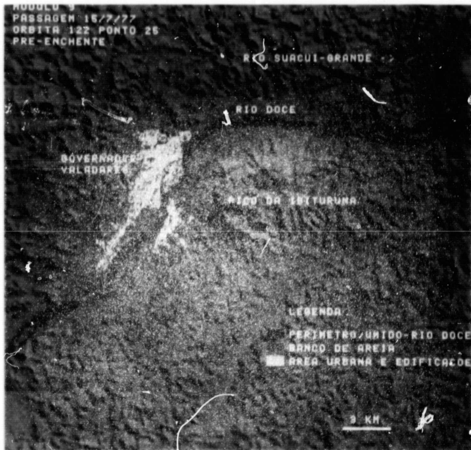
Fig. III.2 - Classificação temática do módulo IX - período de pré-enchente.
