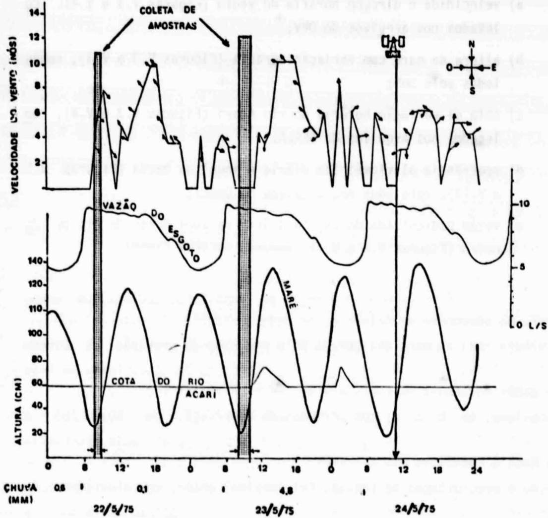
Fig. V.3 - Velocidade do vento, altura da maré e do rio Acari e vazão típica de esgoto para os dias 22, 23 e 24 de maio de 1975.
