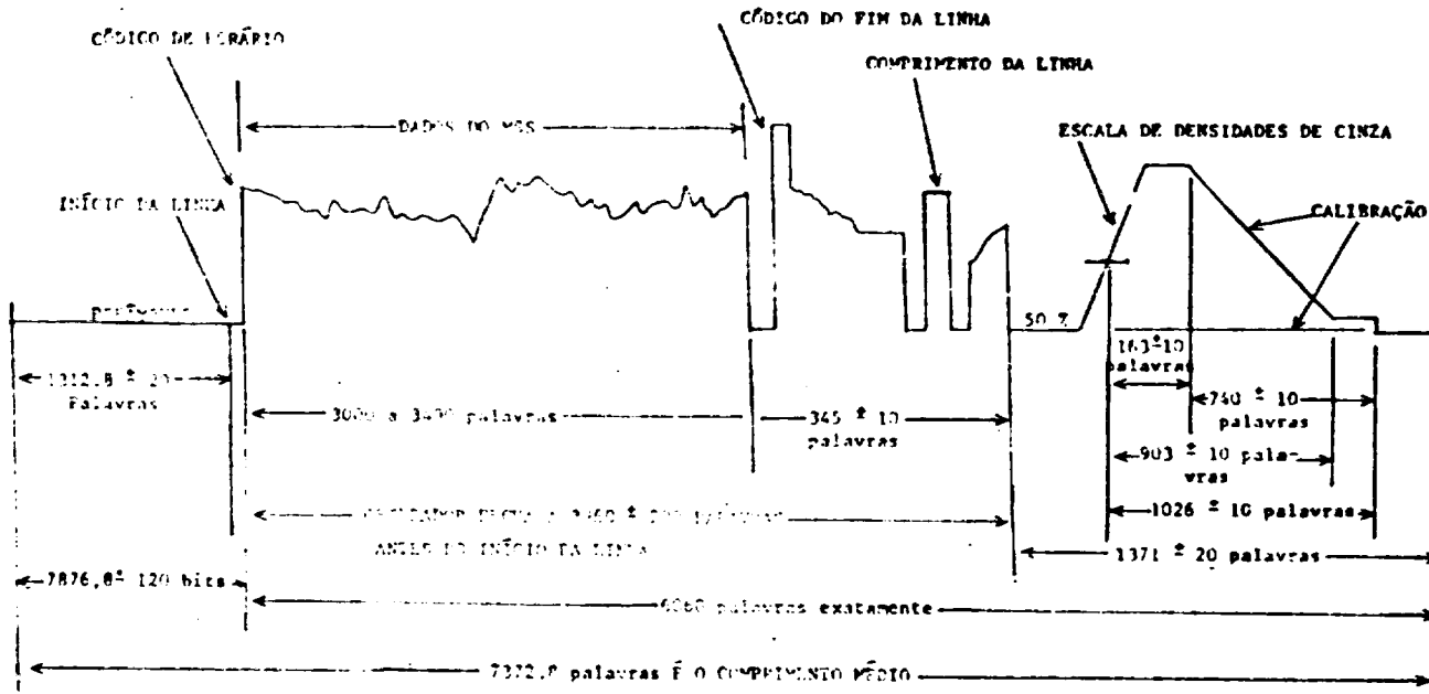
Fig. I.6 - Sequência de dados típica de uma linha de varredura do MSS do LANDSAT. FONTE: NASA (1976), p. C7.
