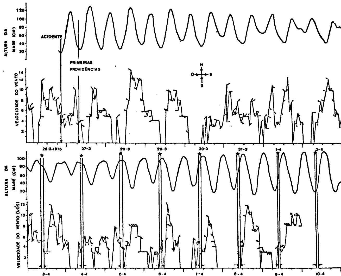
Fig. III.6 - Altura da maré e velocidade do vento nos arredores do acidente com o petroleiro Tarik, após a ocorrência deste (baseado em dados de Coelho e Cunha, 1975, p.232-239; DHN e DPV).
