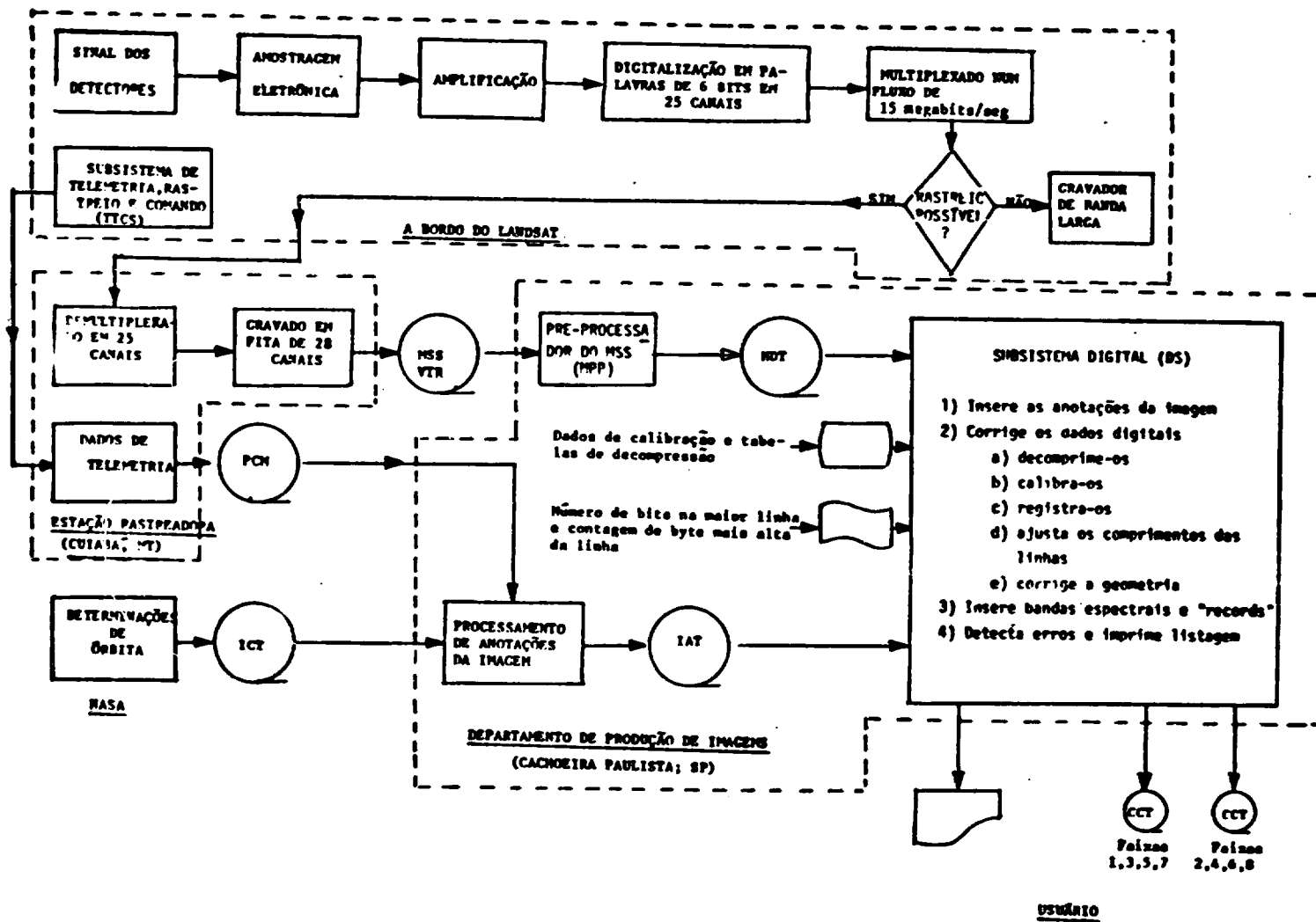
Fig. I.7 - Diagrama de fluxo de processamento de geração de fitas CCT a partir de dados do MSS do LANDSAT.
