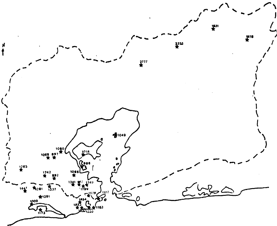
Fig. V.5 - Precipitação de chuvas (em mm) na bacia em 1975. FONTE: SERLA (1979), p. 21 - 602.
