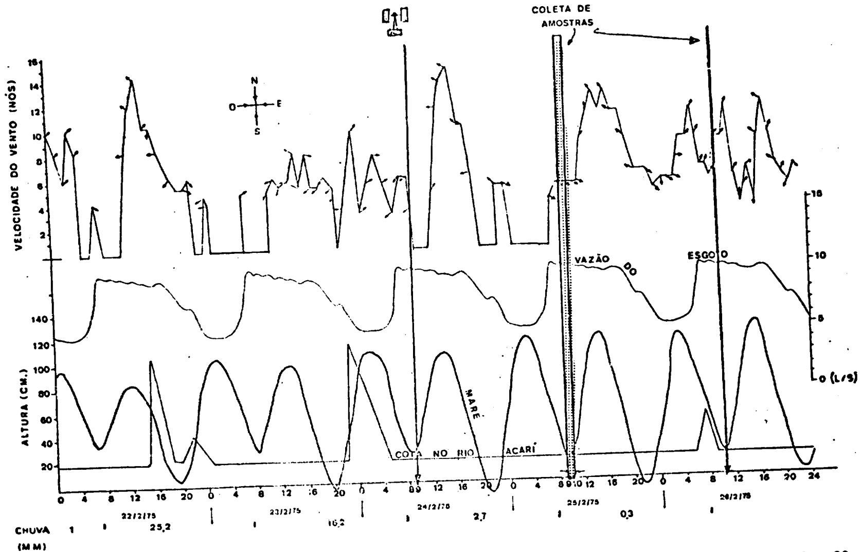
Fig. V.4 - Velocidade do vento, altura da maré e do rio Acari e vazão típica do esgoto para os dias 22, 23, 24, 25 e 26 de fevereiro de 1975.
