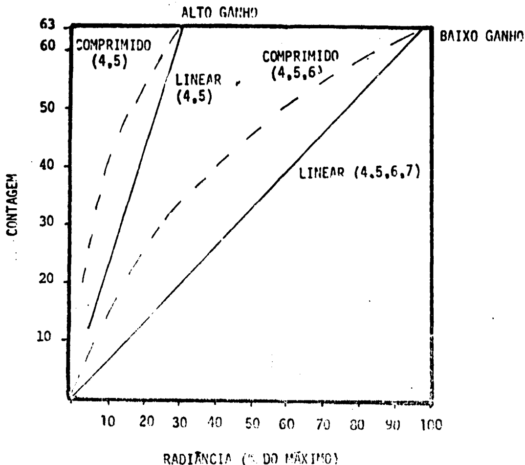
Fig. I.5 - Processamentos analógicos do MSS.
