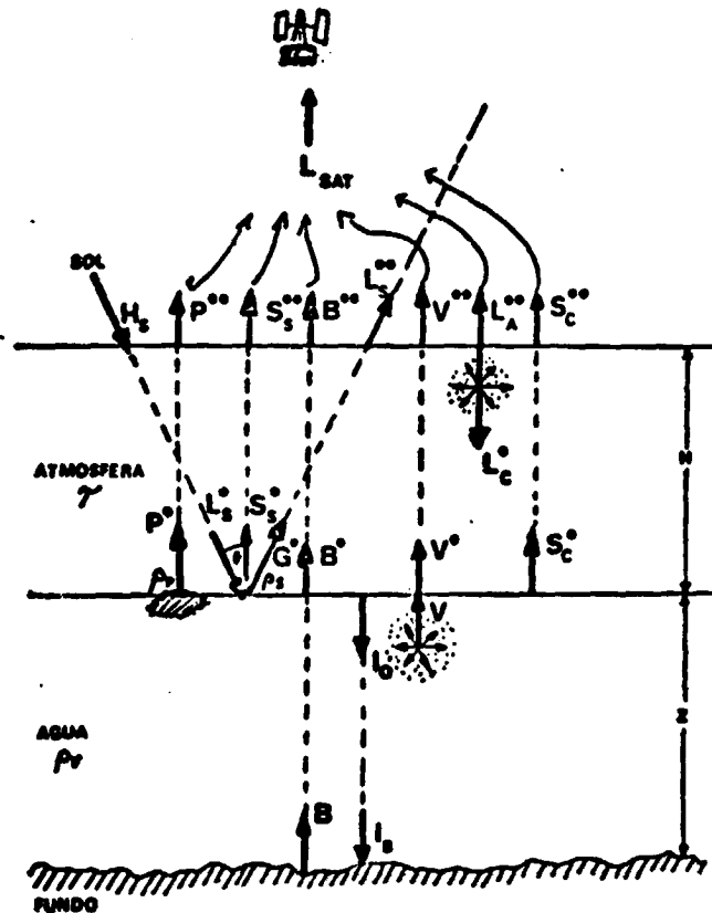
Fig. II.1 - Interação da radiação solar com a atmosfera e a água (baseado em Scherz e Domelen, 1975).
