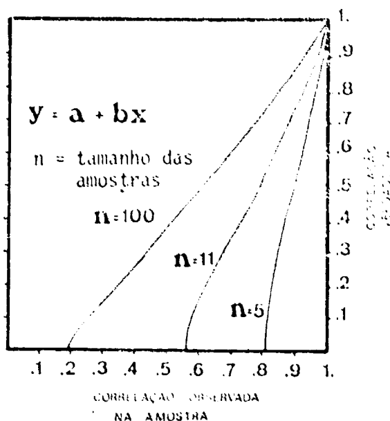
Fig. V.17 - Relação entre o coeficiente de correlação calculado e o verdadeiro, levando-se em consideração que, de cada vinte amostras no Universo, uma está errada.
