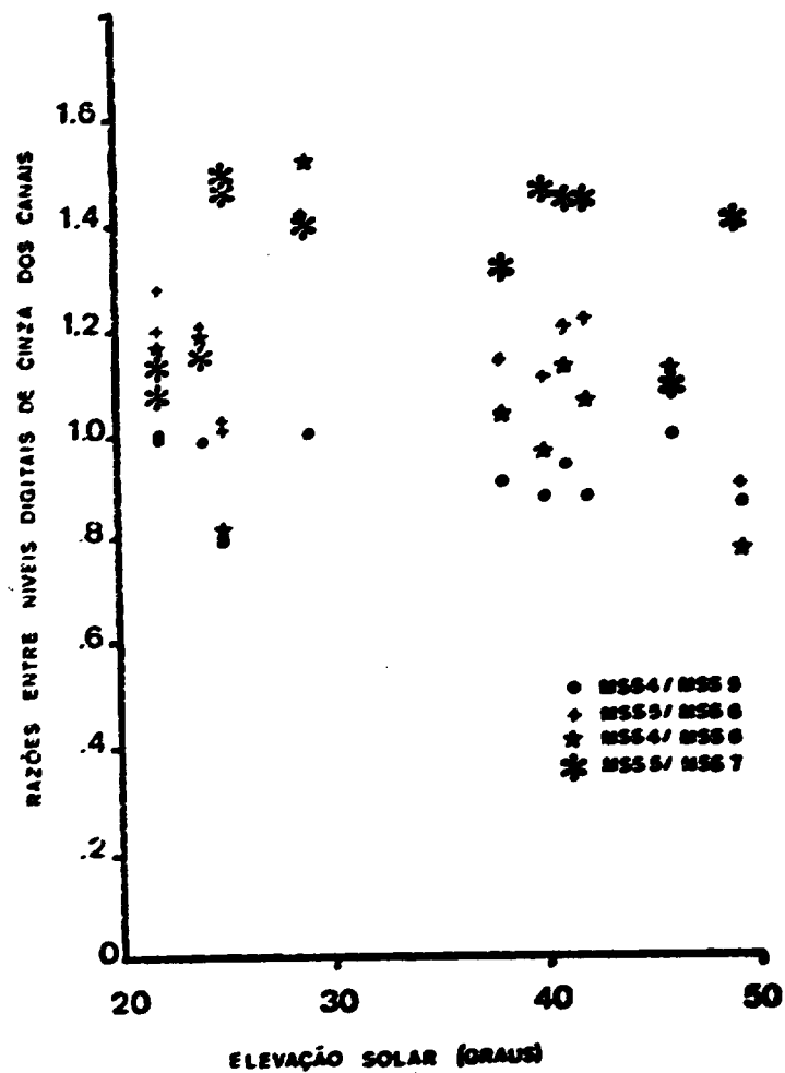
Fig. V.14 - Resultado da aplicação de razões entre faixas adjacentes, utilizando-se os níveis de cinza em imagens com alvos de areia de praia em sobrevôos de diferentes datas ao longo do ano.
