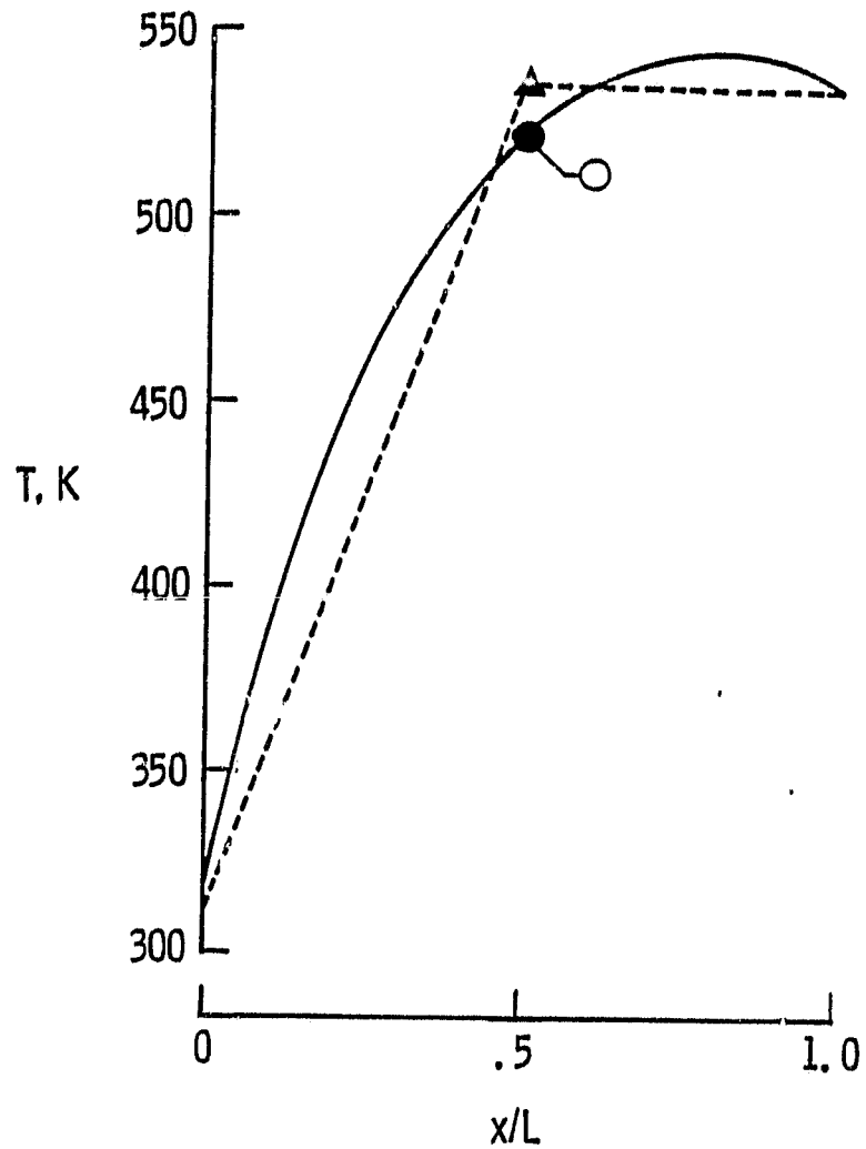
(d) Comparative temperature distributions at t = .30 s.
