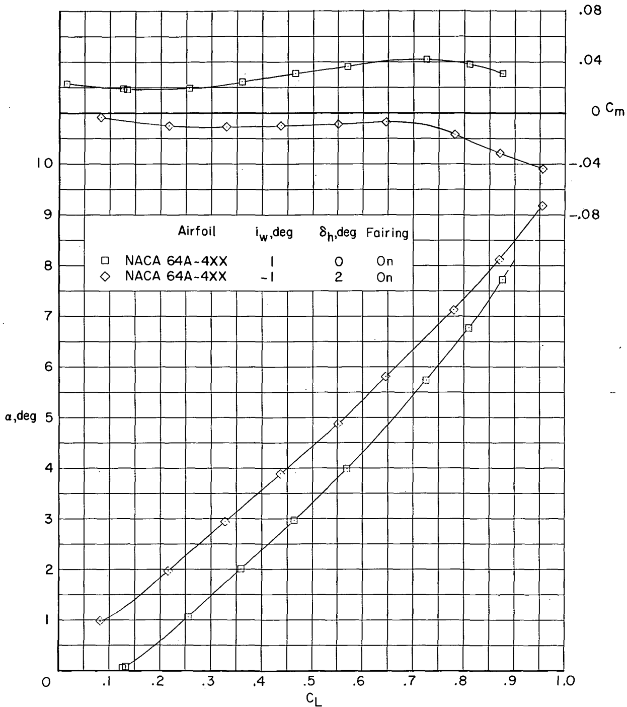
(d) M = 0.80 .
