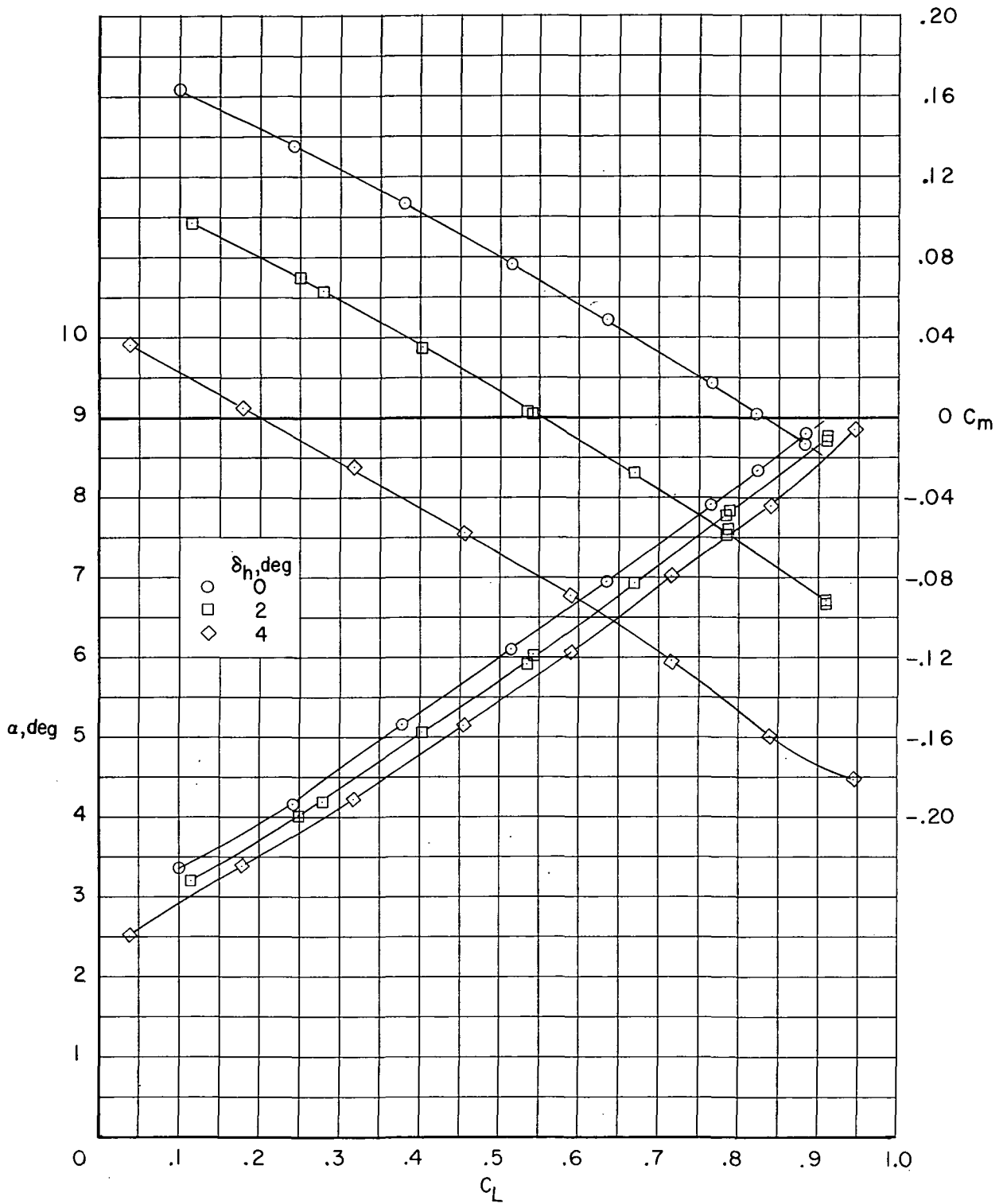
(d) M = 0.91 .
