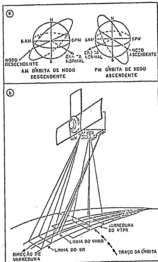
Fig. 4.1 - Órbitas e sensores do satélite NOAA-5
