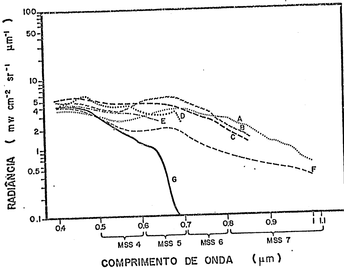
Fig. 2.8 - Radiância espectral calculada com os dados da Figura 2.7, e recebida pelo satélite a 900 km de altura.
