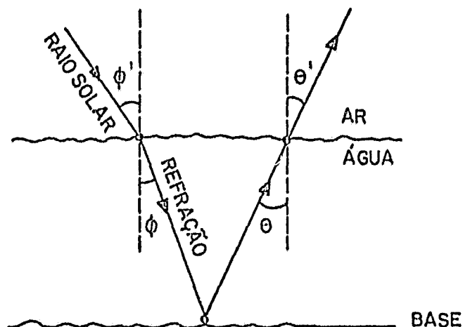
Fig. 2.2 - Raio solar refratado.
