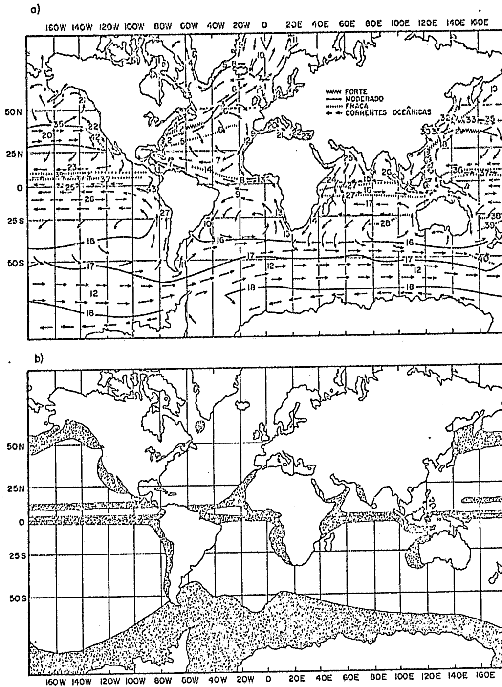
Fig. 4.2 - Posição das correntes e áreas onde ocorrem as ressurgências em escala mundial.
