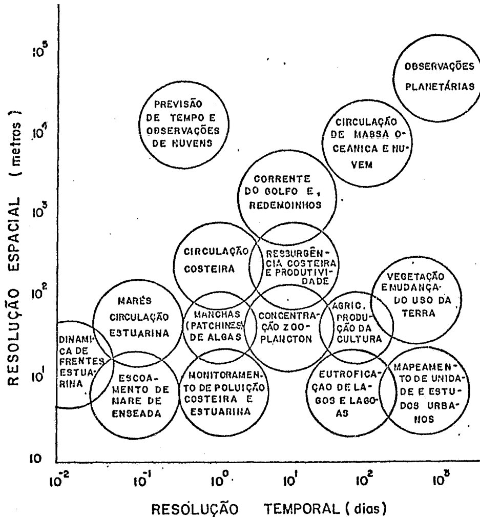
Fig. 3.1 - Resolução temporal e espacial, requeridas para observação de característica oceanográficas, atmosféricas e cobertura de terra.
