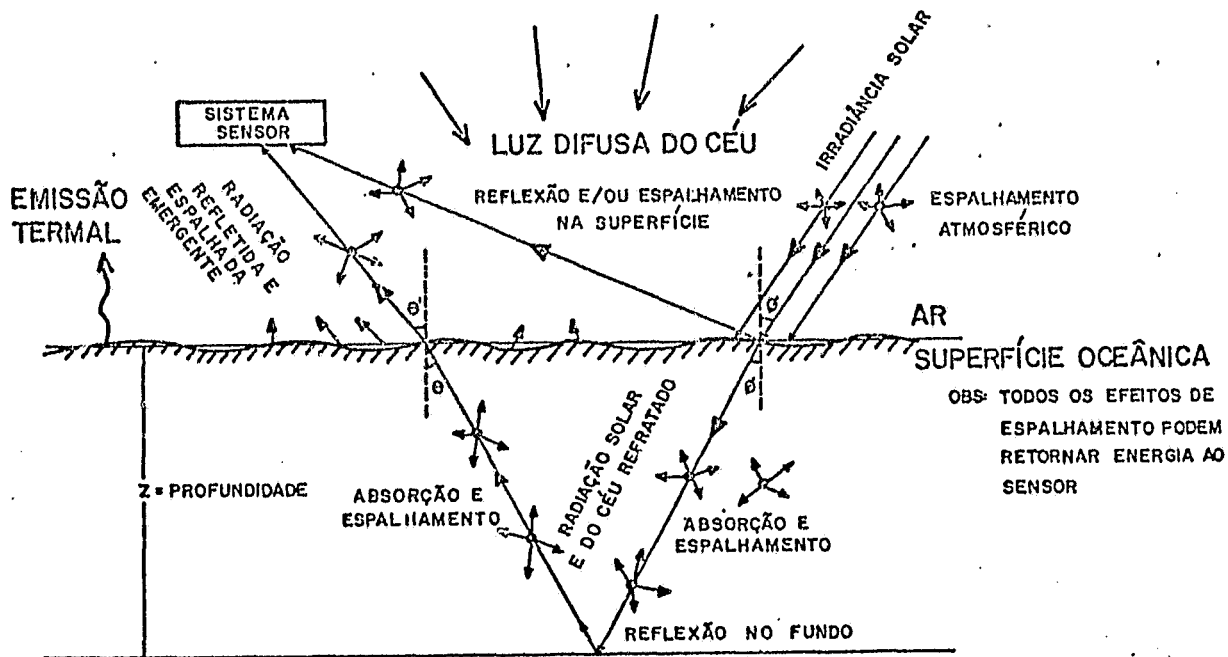
Fig. 1.1 - Processos básicos de interações de um raio solar com a cam da de á gua.
