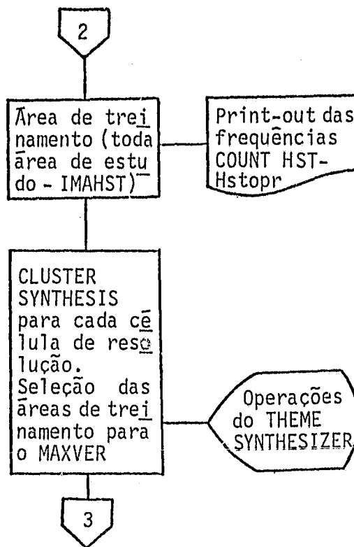
Fig. 3.4 - Fluxograma da seleção das áreas de treinamento para o MAXVER, através de "clustering" ou grupamento.
