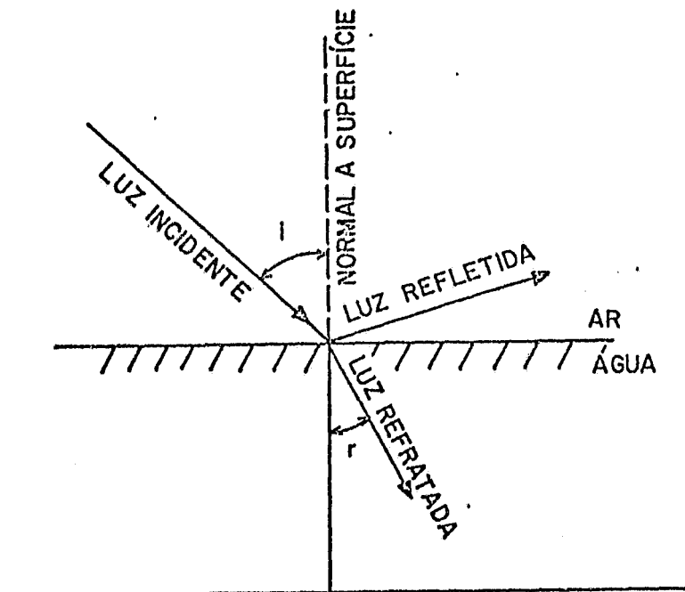
Fig. 2.3 - Feixe de luz incidente, refletido e refratado.
