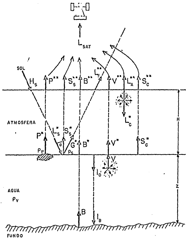
Fig. 2.6 - Interação da radiação solar com a atmosfera e com a água.
