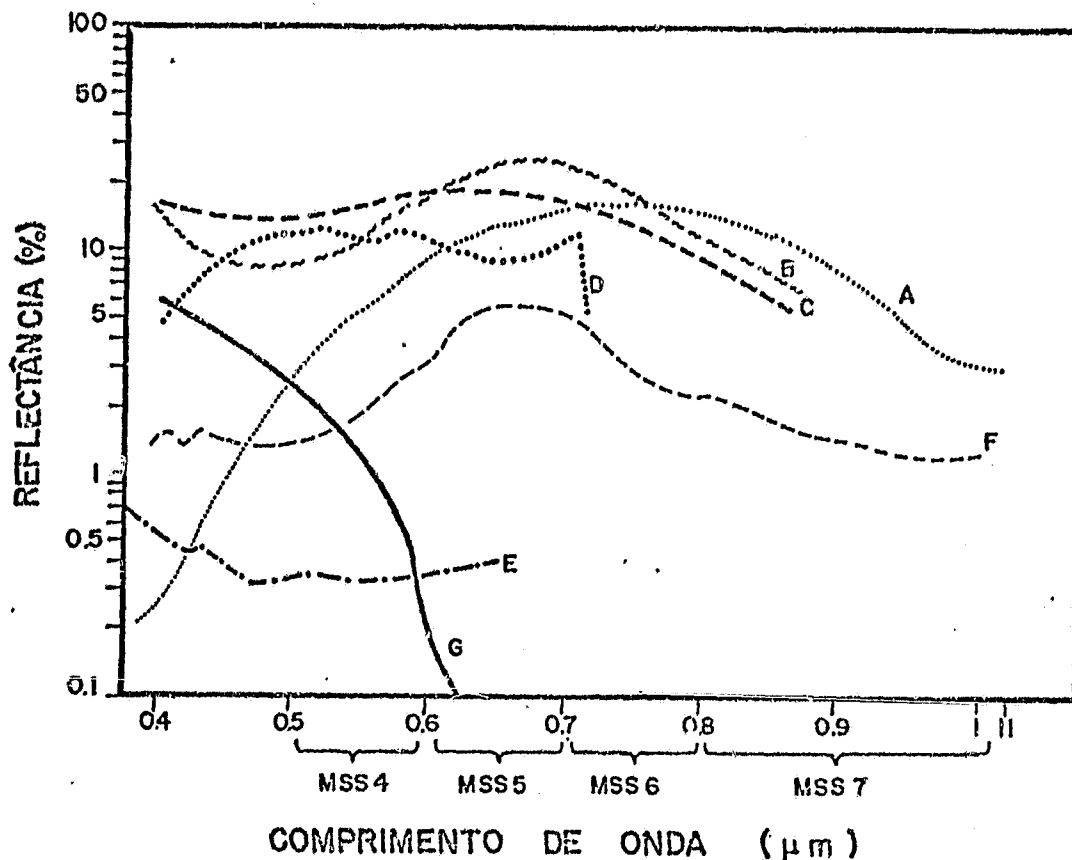
Fig. 2.7 - Reflectância espectral medida em diversos tipos de efluentes industriais e esgotos domiciliares.
