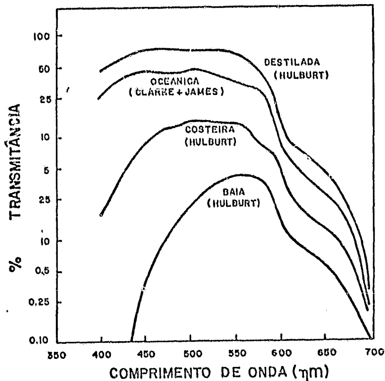
Fig. 2.4 - Transmitância espectral para 10 metros de diversos tipos de água.
