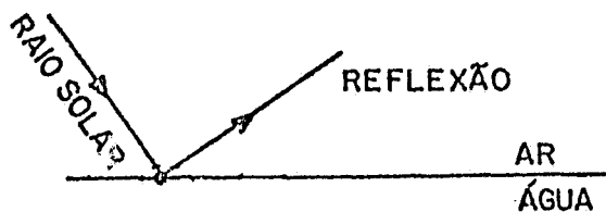
Fig. 2.1 - Raio de sol incidente e refletido.
