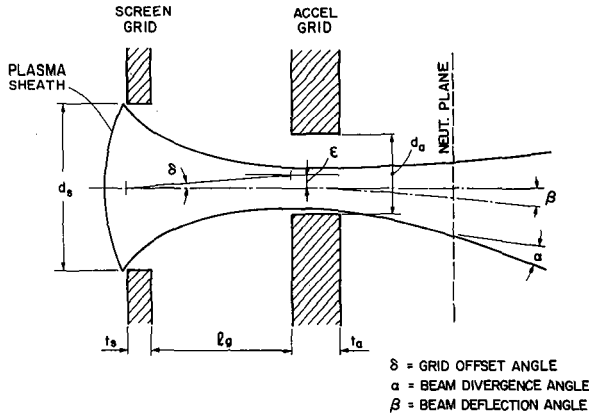
a. BEAMLET NOMENCLATURE
