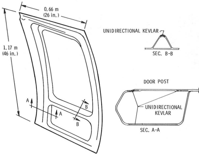
b) Schematic of door
