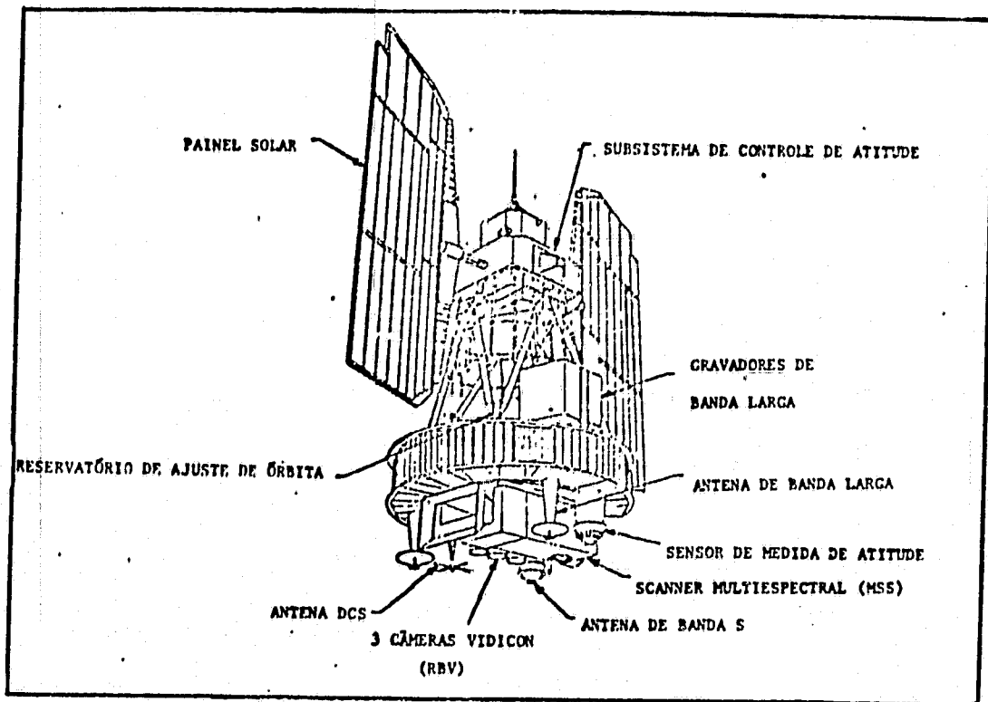
Fig. 2.2 - Configuração do satélite LANDSAT.
