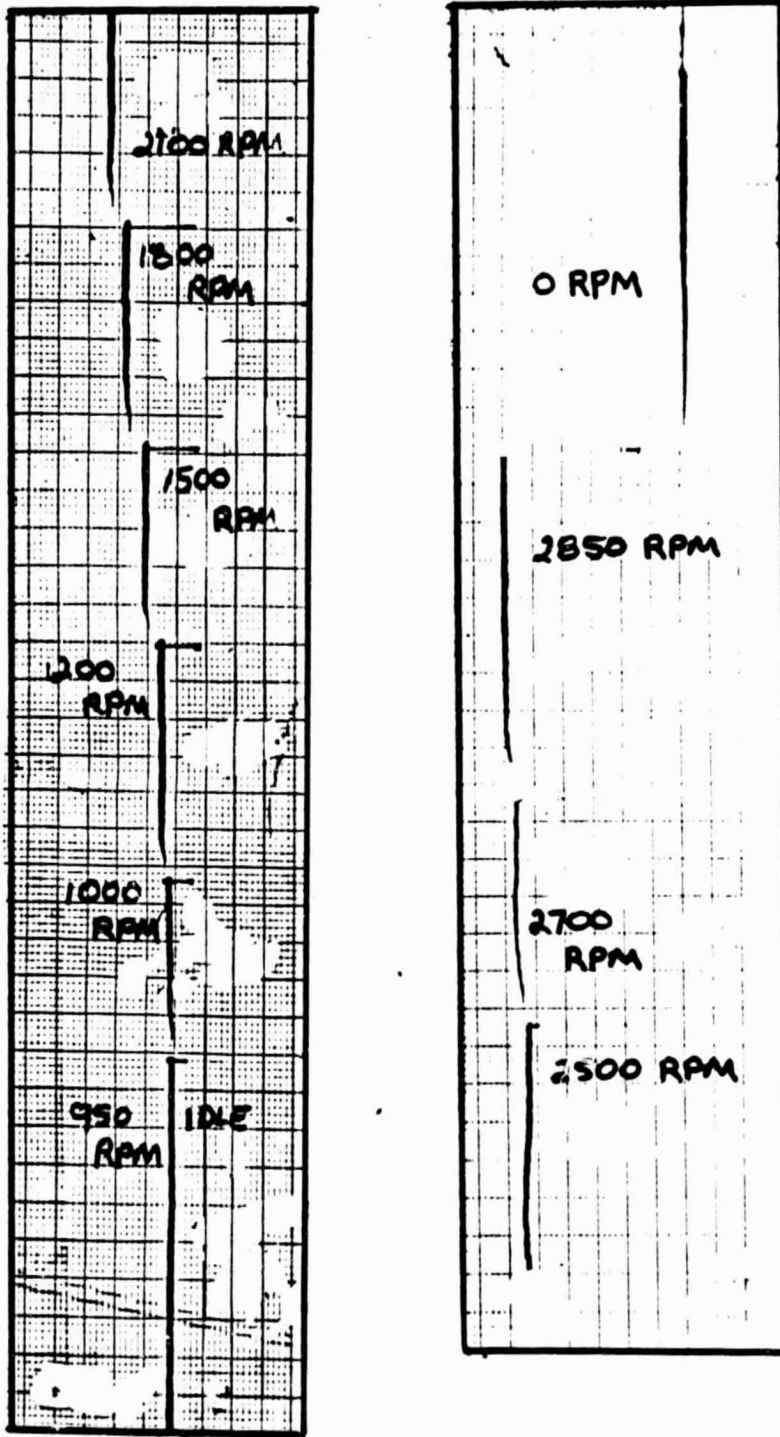
Figure C-6 - Actual Propeller Rpm Calibration Strips
