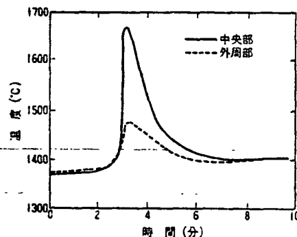
図 6 反応焼結の進行に伴うペレットの温度変化 (10 -4 トールの真空中で加熱、2°C/min、1370°C で電源を断つ)
