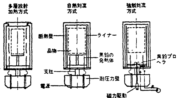
図 8 HIP における作業窯加熱方式の三つの例 (オートクレーブ社)
