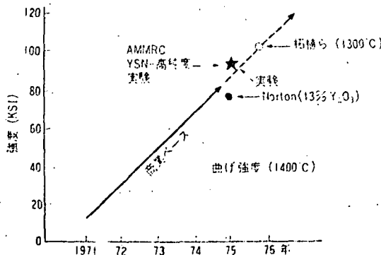
図2 Si 3 N 4 の高温強度改善
