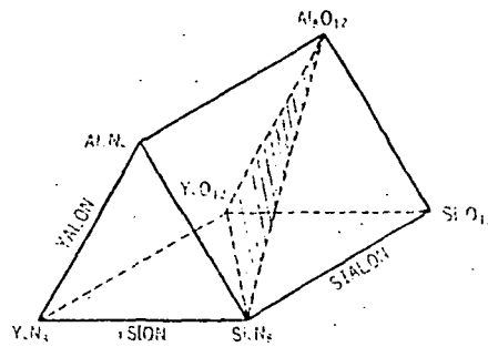
図3 Si 3 N 4 -Y 2 O 3 -Al 2 O 3 系
