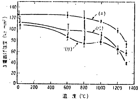
図9 粒界結晶化と強度 ( \text{Si}_3\text{N}_4 -5wt% \text{Y}_2\text{O}_3 -2wt% \text{Al}_2\text{O}_3 ) A: 結晶化, B, C: 非結晶化 9)
