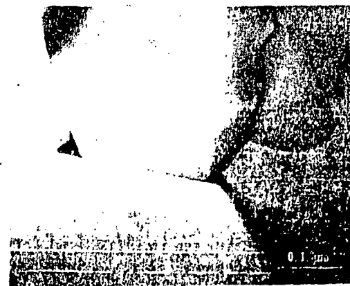
図1 ホットプレス Si 3 N 4 の微細構造 (Si 3 N 4 -5 wt% Y 2 O 3 -2 wt% Al 2 O 3 )
