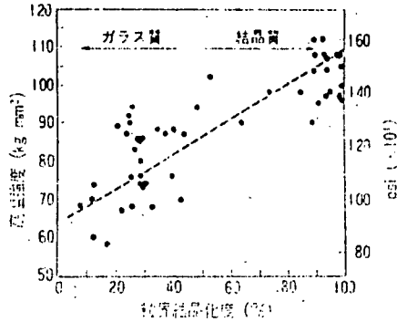
図10 高温強度に及ぼす粒界結晶化の影響 9)
