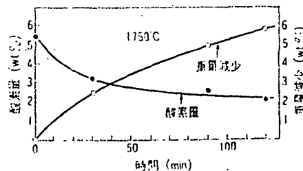
図4 Si 3 N 4 -5 wt% Y 2 O 3 -2 wt% Al 2 O 3 成形体の AlN 粉中の熱処理に伴う変化
