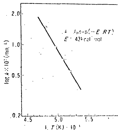
図 7 結晶化のアレニウスプロット
