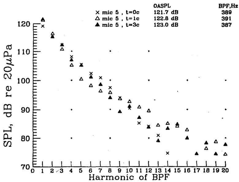
(d) inplane ( \theta = 0^\circ ), microphone 5.
