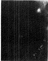
PELE (IO)
