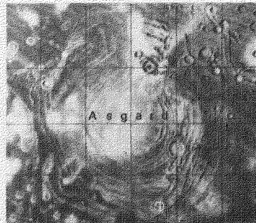
ASGARD (CALLISTO)
