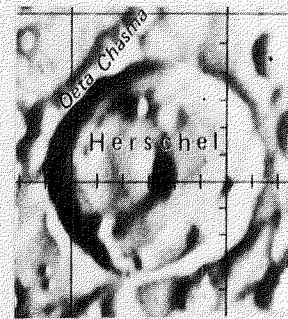
HERSCHEL (MIMAS)
