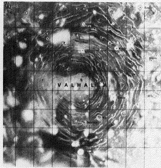
VALHALLA (CALLISTO)
