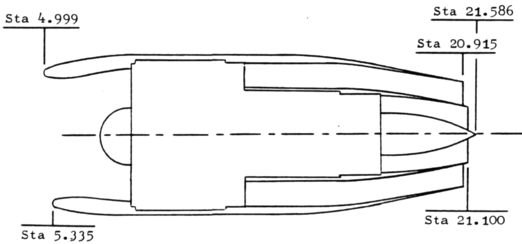
E 3 Nacelle
