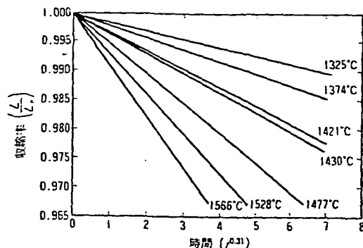
図 2(a) 等温収縮と時間の関係
