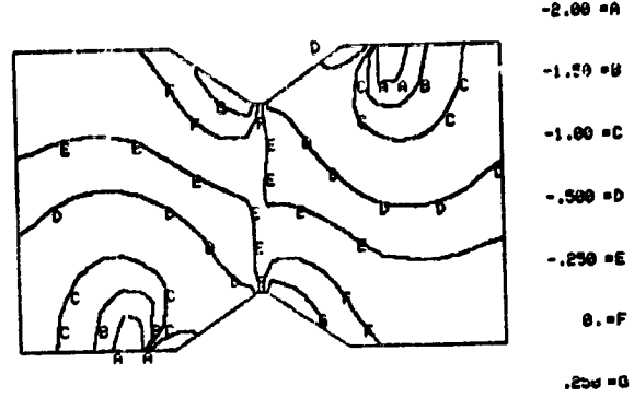
b) Increment 4, 57.1 MPa (8.28 ksi)
