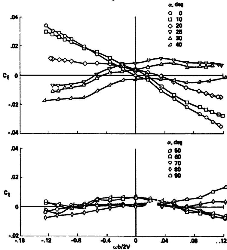
(b) Rolling-moment coefficient.
