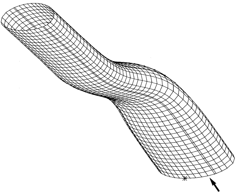
Simple (ellipse)
