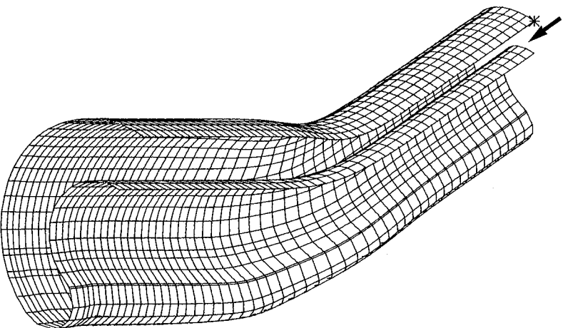
Complex (saddlemanulus)
