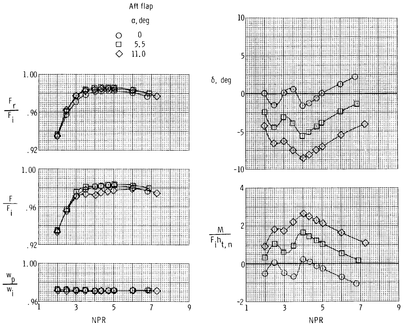
(d) Configuration A3FS, \delta_v = -4.15^\circ .
