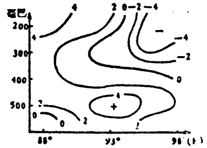
图 5b 1979 年 6 月 8 日 20 时 11°N 涡度 ( 10^{-5} \text{秒}^{-1} ) 垂直分布
