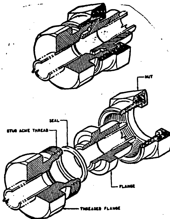
Figure 28. Gamah Edge Seal
