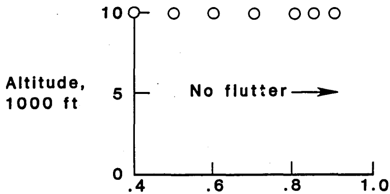
(b) Initial decoupler pylon.
